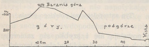
Przekrój przez Podgórze i przez Beskid Śląski (podz. dług. 1:750.000, podz. wys. 1:50.000).
