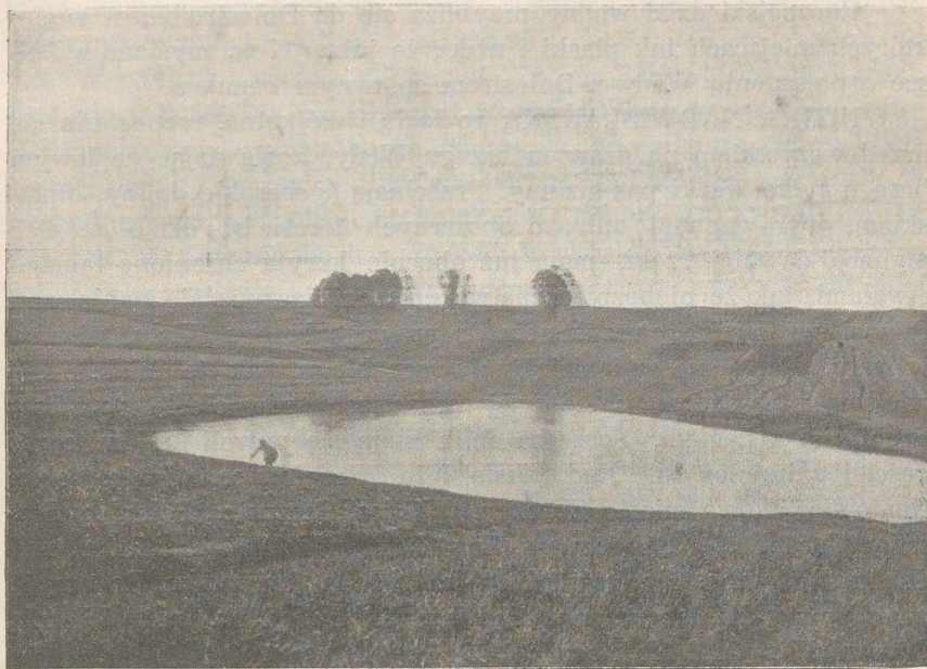
Jeziorko w Szkle na podłożu glin dyluwialnych. Z powodu zawartości siarki występuje tu flora i fauna właściwa wodom siarczanym.
