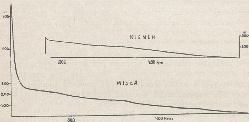
Spadek Wisły, rzeki górsko-nizinnej i Niemna, rzeki nizinnej.
