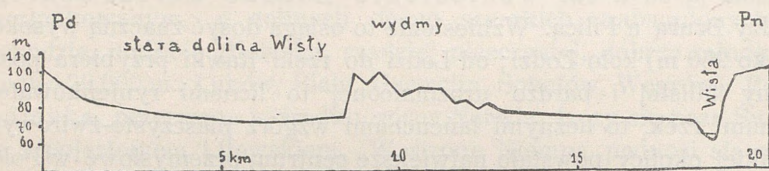
Przekrój przez dolinę Wisły poniżej Warszawy.
