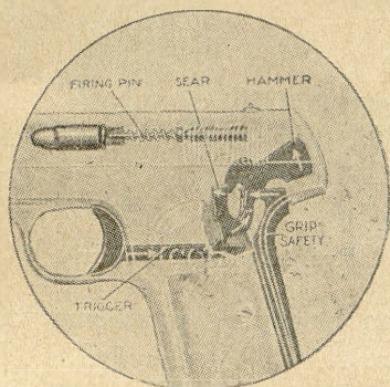
Rys. 9. Bezpiecznik w ręczce Colta.
