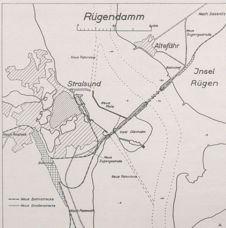
Der Rügendamm bei Stralsund. 1936 fertiggestellt.
