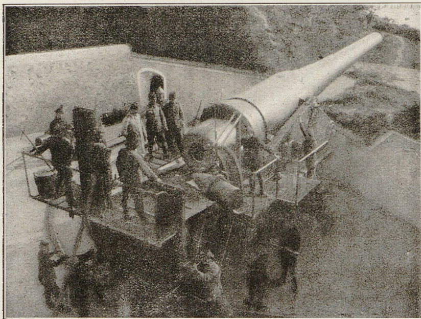
Deutsche und türkische Mannschaften am 35,5 cm-Geschütz bei Rumeli Kavat.
