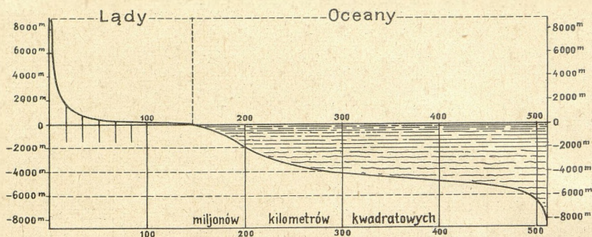
Ryc. 13. Krzywa hipsograficzna.
