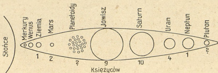
Ryc. 6. Planety w porządku ich oddalenia od słońca i według wielkości. Księżyc planet.
