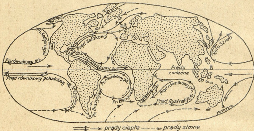
Ryc. 36. Schemat prądów morskich.
