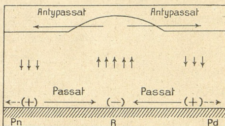
Ryc. 33. Krążenie powietrza na ziemi w pobliżu równika.
