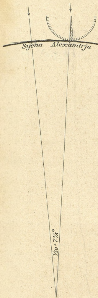
Ryc. 1. Pomiar wielkości ziemi przez Eratostenesa.
