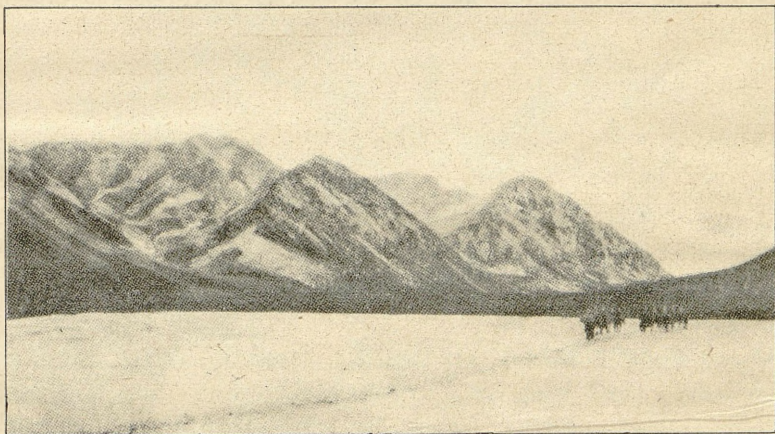
Ryc. 97. Góry Czerskiego w Syberji wschodniej.
