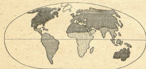
1. Notogeia 2. Neogeia 3. Arctogeia a) kraina ełjopska b) kraina orientalna c) kraina palear- ktyczna d) kraina nearktyczna
