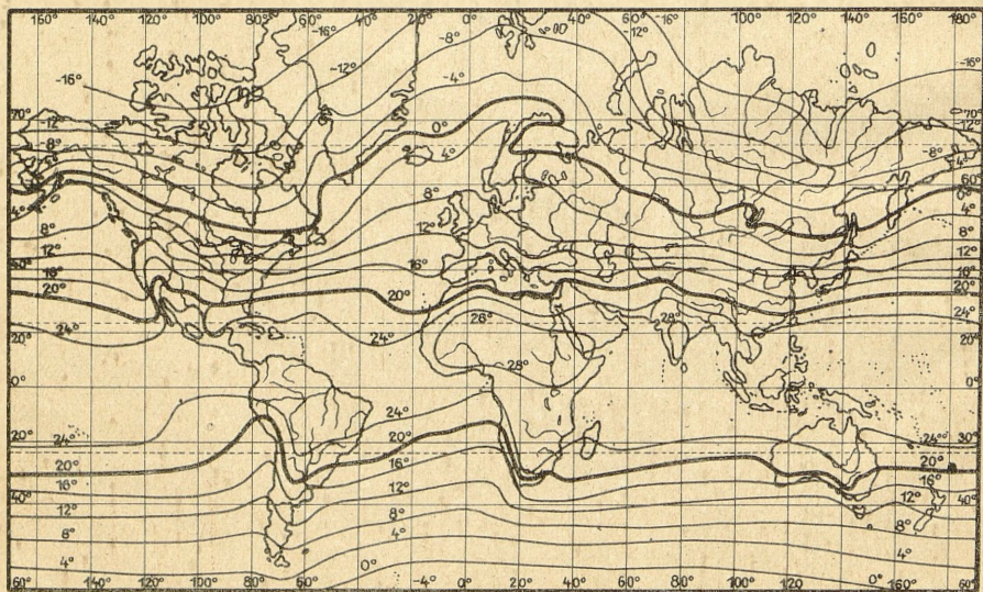
Ryc. 27. Izoterm y roczne.
