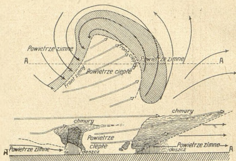
Ryc. 31. Na górnej rycinie widzimy (w rzucie poziomym), jak powietrze ciepłe na powierzchni ziemi napływa do środka cyklonu od południowego zachodu. Dolna rycina daje przekrój: A A przez cyklon i wyjaśnia powstanie deszczu.
