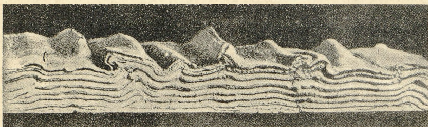
Ryc. 21. Proces fałdowania.
