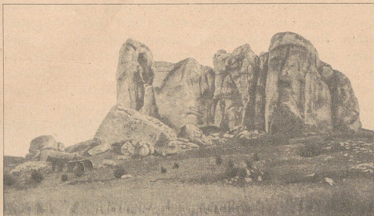
Ryc. 118. Skały wapienne Grzbietu Krakowsko-Wieluńskiego.
