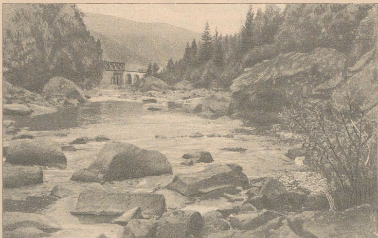
Ryc. 103. Piękny krajobraz doliny Prutu.
