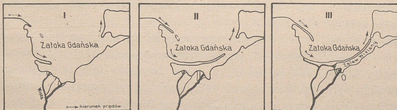
Ryc. 222. Schemat powstawania mierzei.
