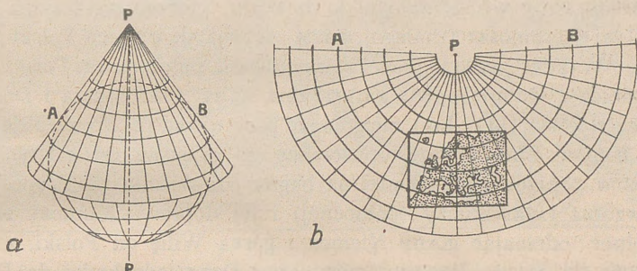
Ryc. 2 a — stożek nałożony na kulę; 2 b — pobocznica stożka rozplaszczona i układ południków i równoleżników w siatce stożkowej. W ramce mapa Europy.
