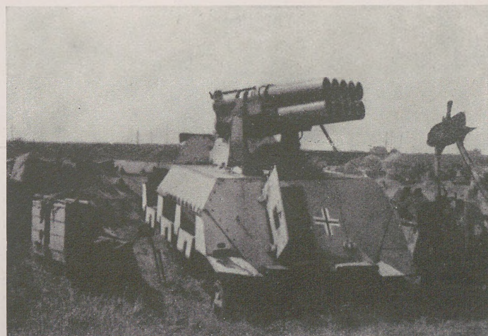
Wielolufowe moździerze strzelały w rejon zniszczonych mostów, utrudniając przeprawę. These ten-barrelled mortars covered the destroyed bridges. They didn't make river crossings any easier.
