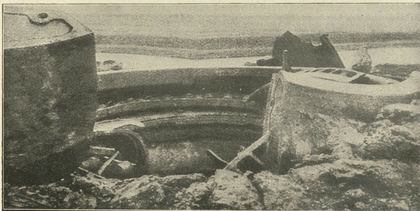
Fort Wavre-Ste. Catherine Ein durch 42-cm-GeschöÙ zerstörter 15-cm-Panzerturm und Blick auf den Wassergraben.
