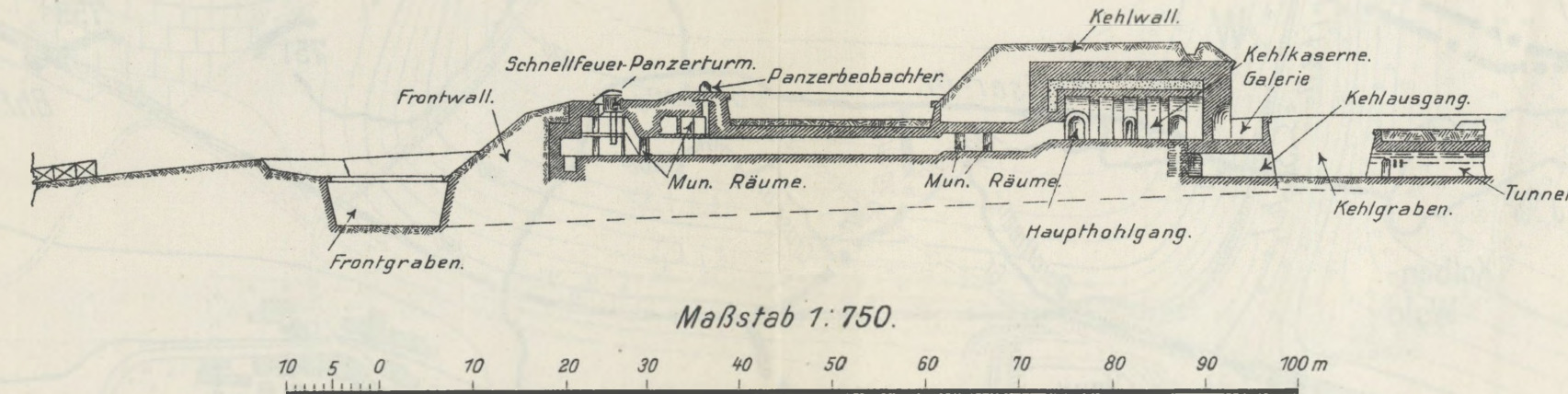
Querschnitt durch das Fort von Nordost nach Südwest (a-b).
