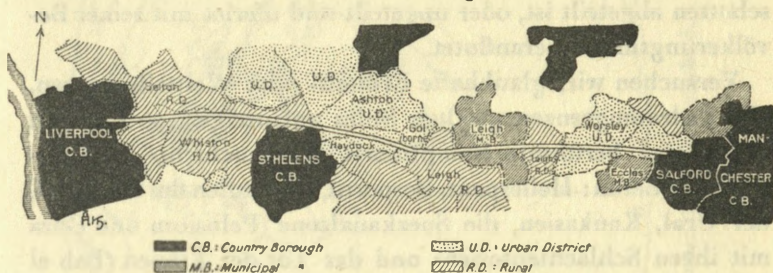
10. Stadt- und Landgrenzen im Verkehrsdruck: die Straße Manchester—Liverpool.
