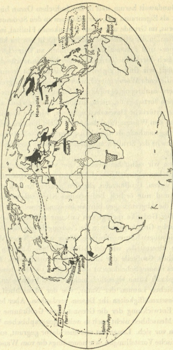
11. Kampzonen der Kontinentscheiden.
