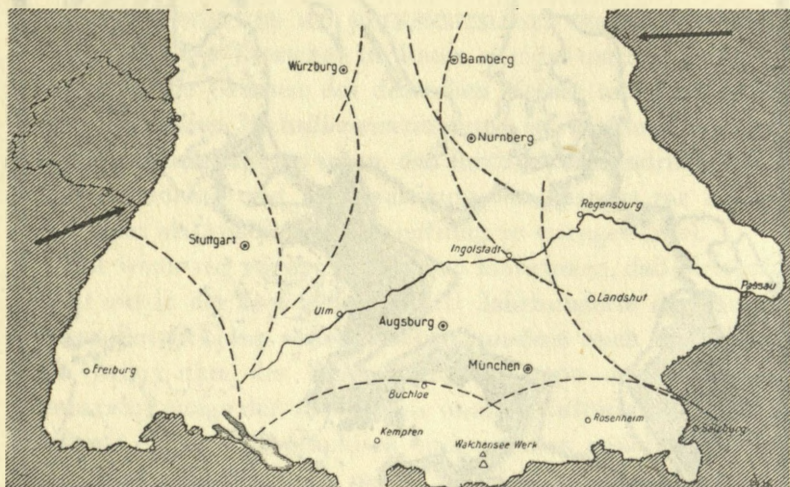
28. Fremdfeuerbereich über Süddeutschland.
