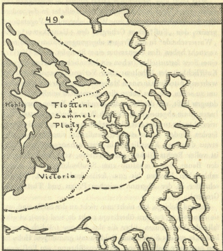
5. Die Juan de Fuca-Grenze.
