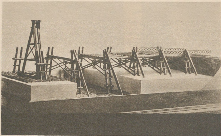
MAKIETA MOSTU CEZARA NA RENIE (St. Germain en Laye)
