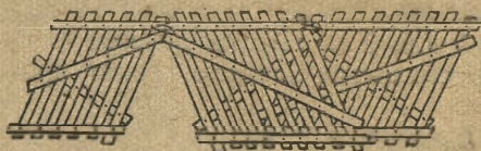
Рис. 20. Наклонная установка плечных щитов
