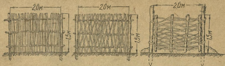
Рис. 18. Типы хворостяных щитов
