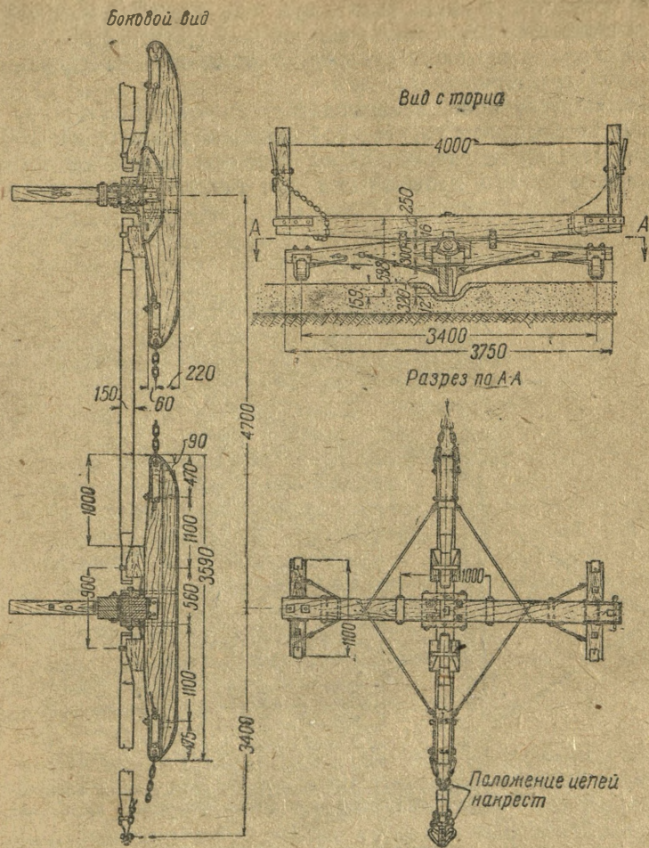
Рис. 29. Тракторные однополосные сани одноколейной железной дороги
