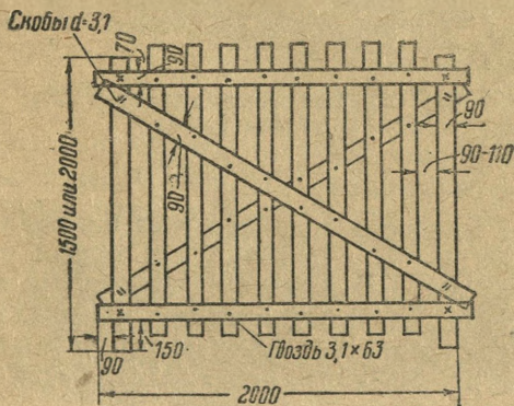
Рис. 19. Планочный щит
