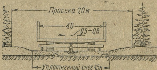
Рис. 25. Одноколейная ледяная дорога на одну полосу движения
