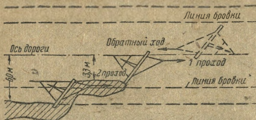
Рис. 21. Работа одноотвального тракторного треугольника при толщине снега до 40 см
