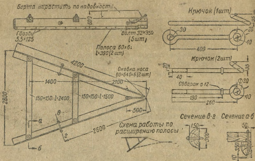
Рис. 6. Конный треугольник из пластин
