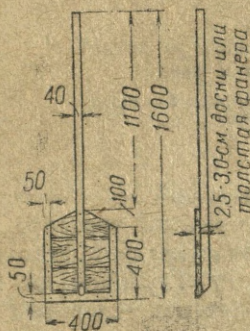
Рис. 9. Деревянная снеговая лопата.
