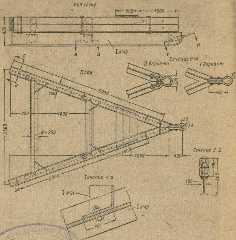
Рис. 14. Металлический тракторный двухотвальный треугольник
