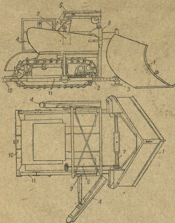
Рис. 12. Тракторный плужный двухотвальный снегоочиститель ДАК-2:
