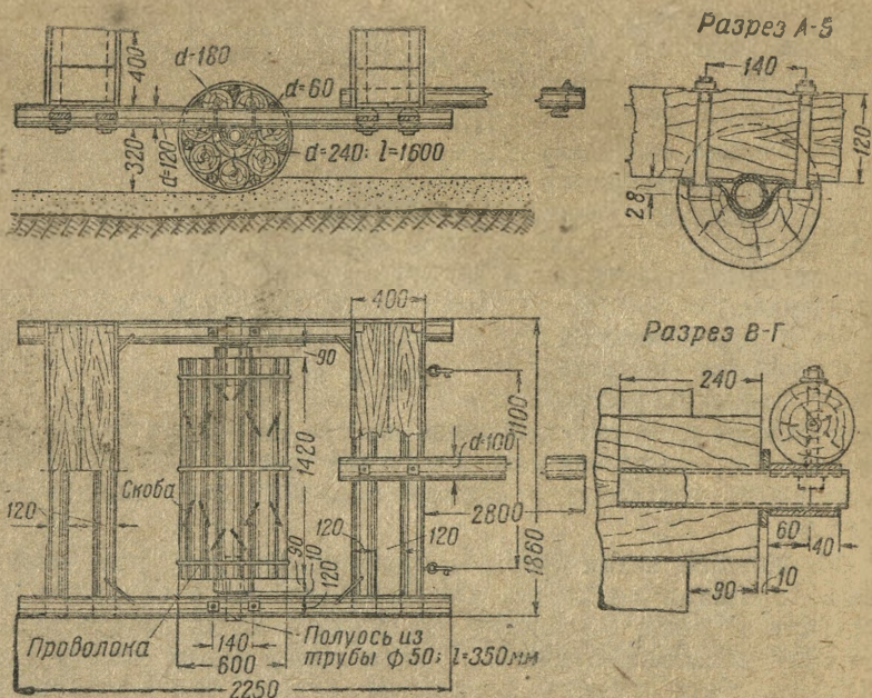
Рис. 4. Конный каток
