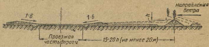
Рис. 17. Снеговой вал, его расположение относительно дороги и последующее наращивание высоты лапником
