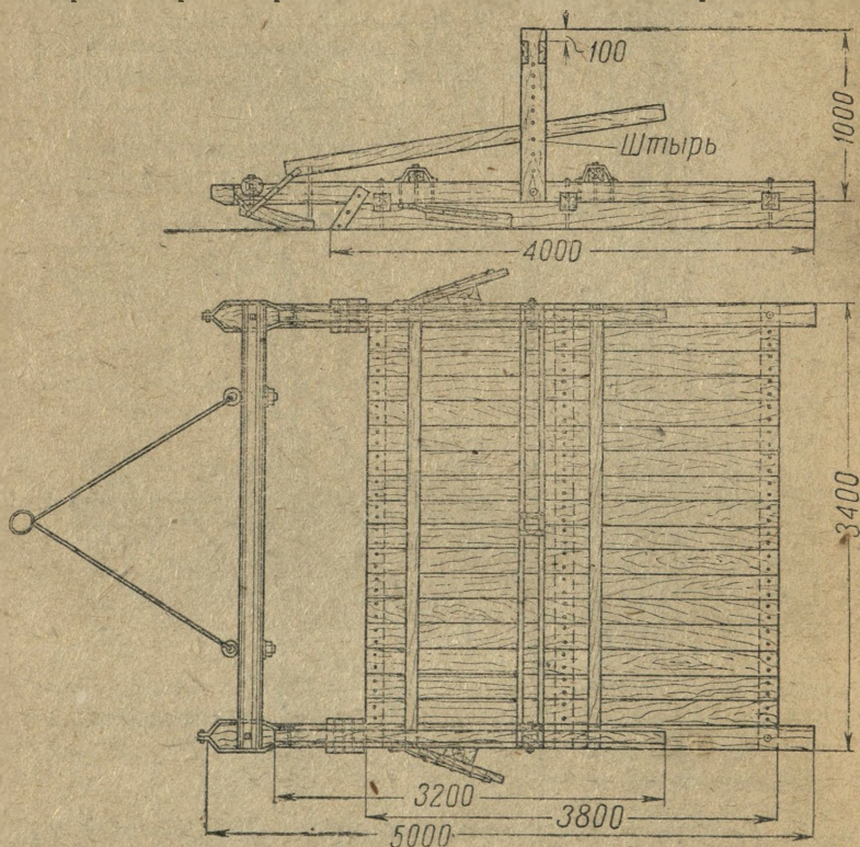
Рис. 30. Колеерез для двухколейной тракторной ледяной дороги
