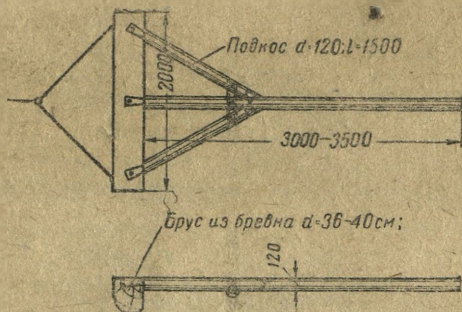
Рис. 3. Конная волокуша
