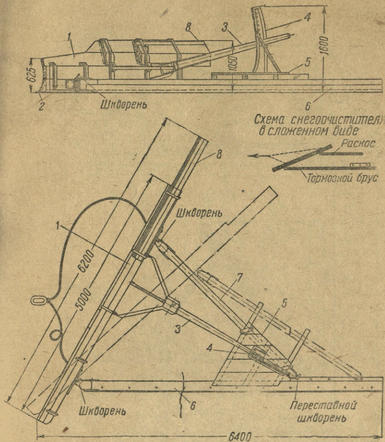
Рис. 15. Тракторный одноотвальный снегоочистительный треугольник с изменяемой шириной захвата:
