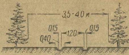
Рис. 27. Ледяная дорога для конной тяги на земляном основании
