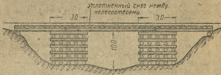
Рис. 8. Мост на клетках
