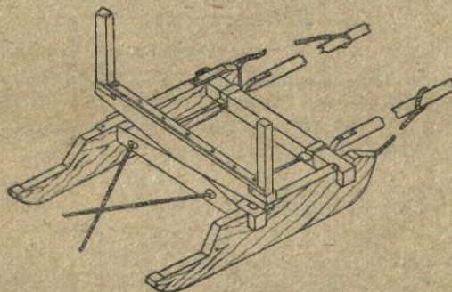
Рис. 28. Подсанок двухколейных саней конной тяги. Сани состоят из двух одинаковых подсанков
