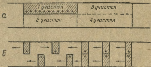
Рис. 11. Схема организации работ по ручной очистке дороги от снега и льда:
