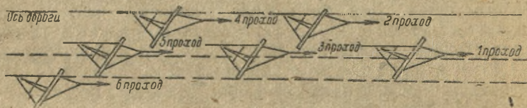
Рис. 22. Работа одноотвального тракторного треугольника при толщине снега свыше 40 см методом послойной очистки снега
