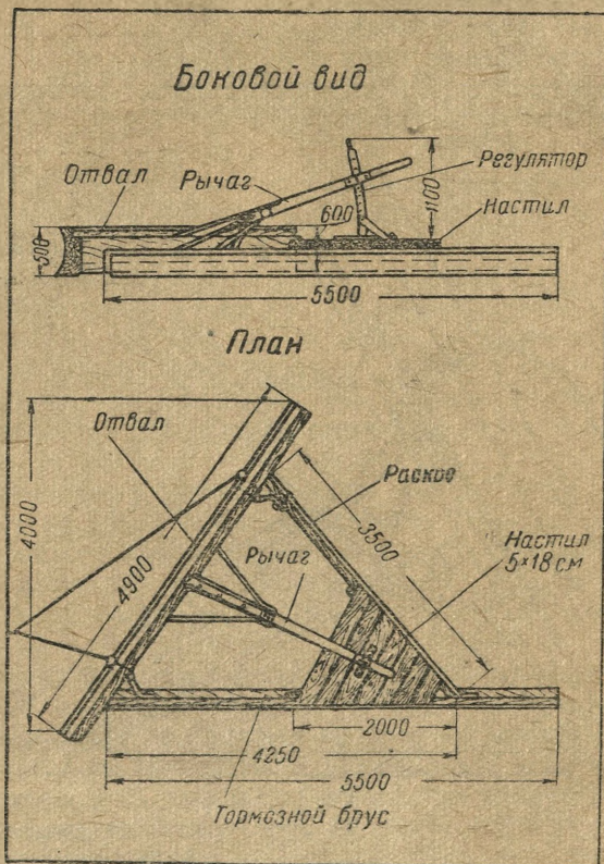
Рис. 16. Тракторный одноотвальный снегоочистительный треугольник с неизменяемой шириной захвата. (Детали снегоочистителя см. на стр. 27, 28, 29 и 30)
