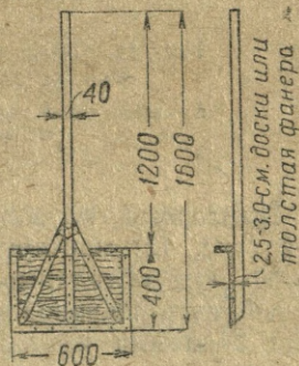
Рис. 10. Деревянный скребок
