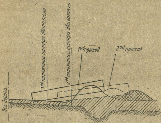
Рис. 24. Схема разравнивания валов одноотвальным треугольником
