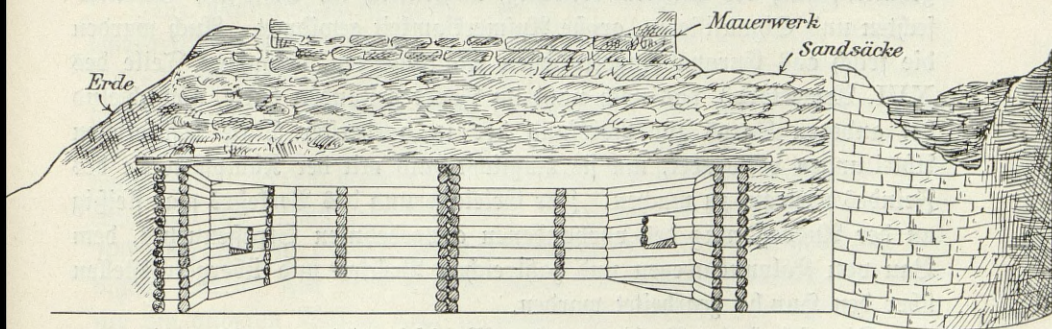
Schnitt A-B.
