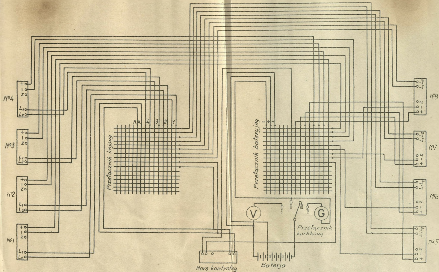
Ryc. 8. Układ połączeń sali aparatuwej morsa.
