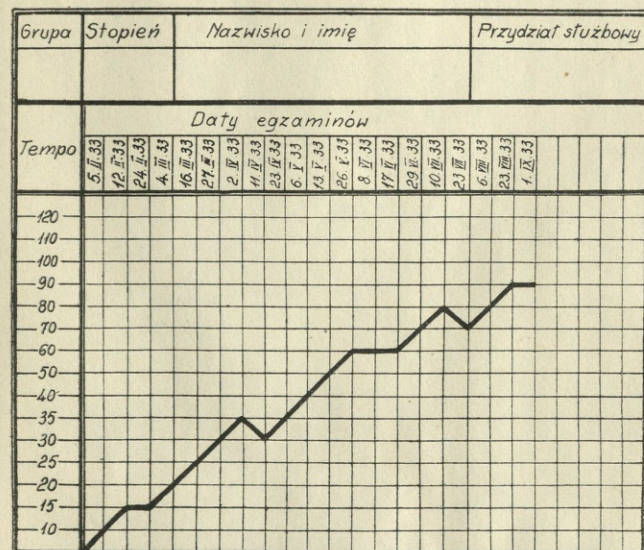
Ryc. 1. Przykład wykresów z odbioru słuchowego.
