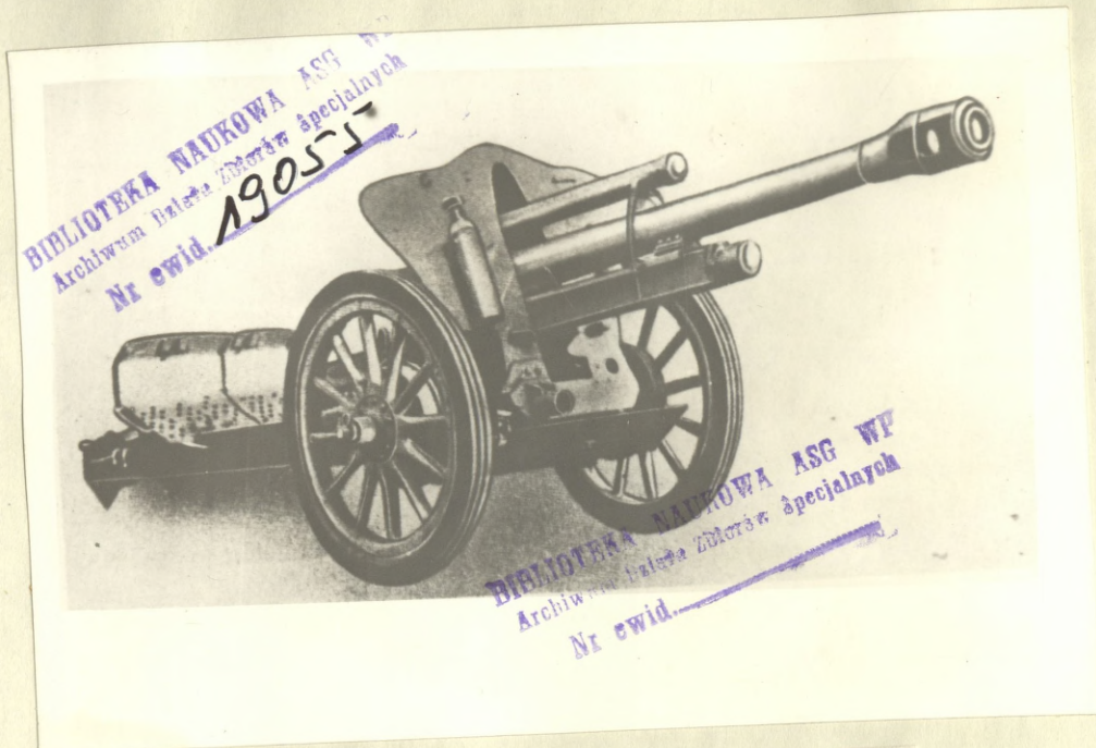
28. N. 10,5 cm haubica polowa 18 ML/28
