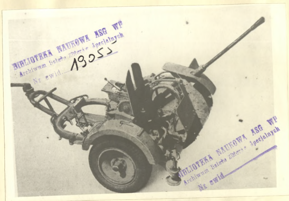
34. N. 2 cm działko przeciwlotnicze
