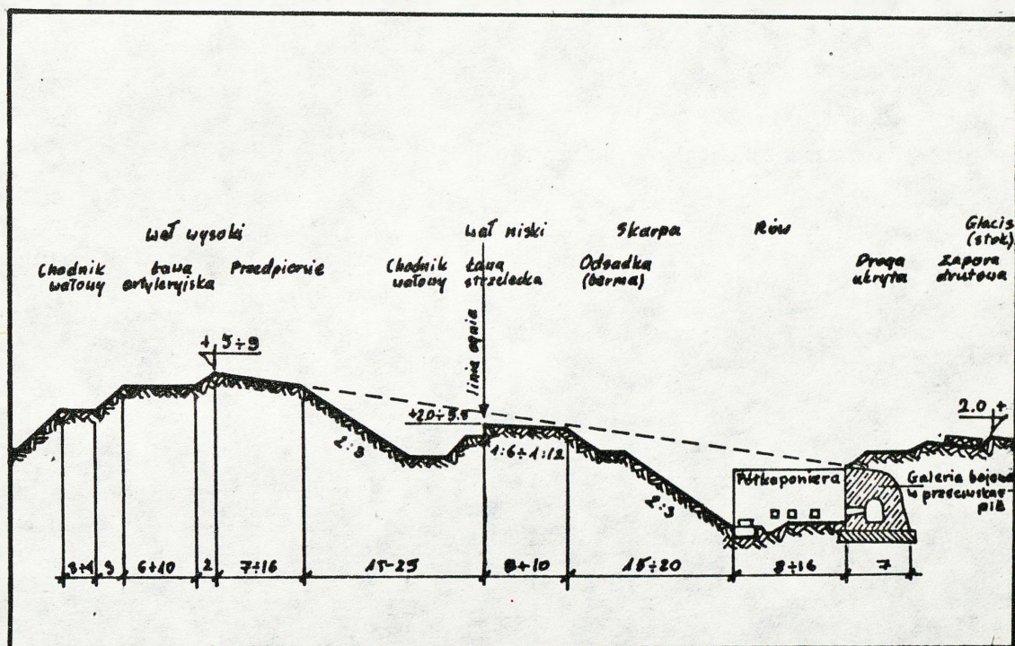
Przekrój poprzeczny przez wały i rów forteczny
