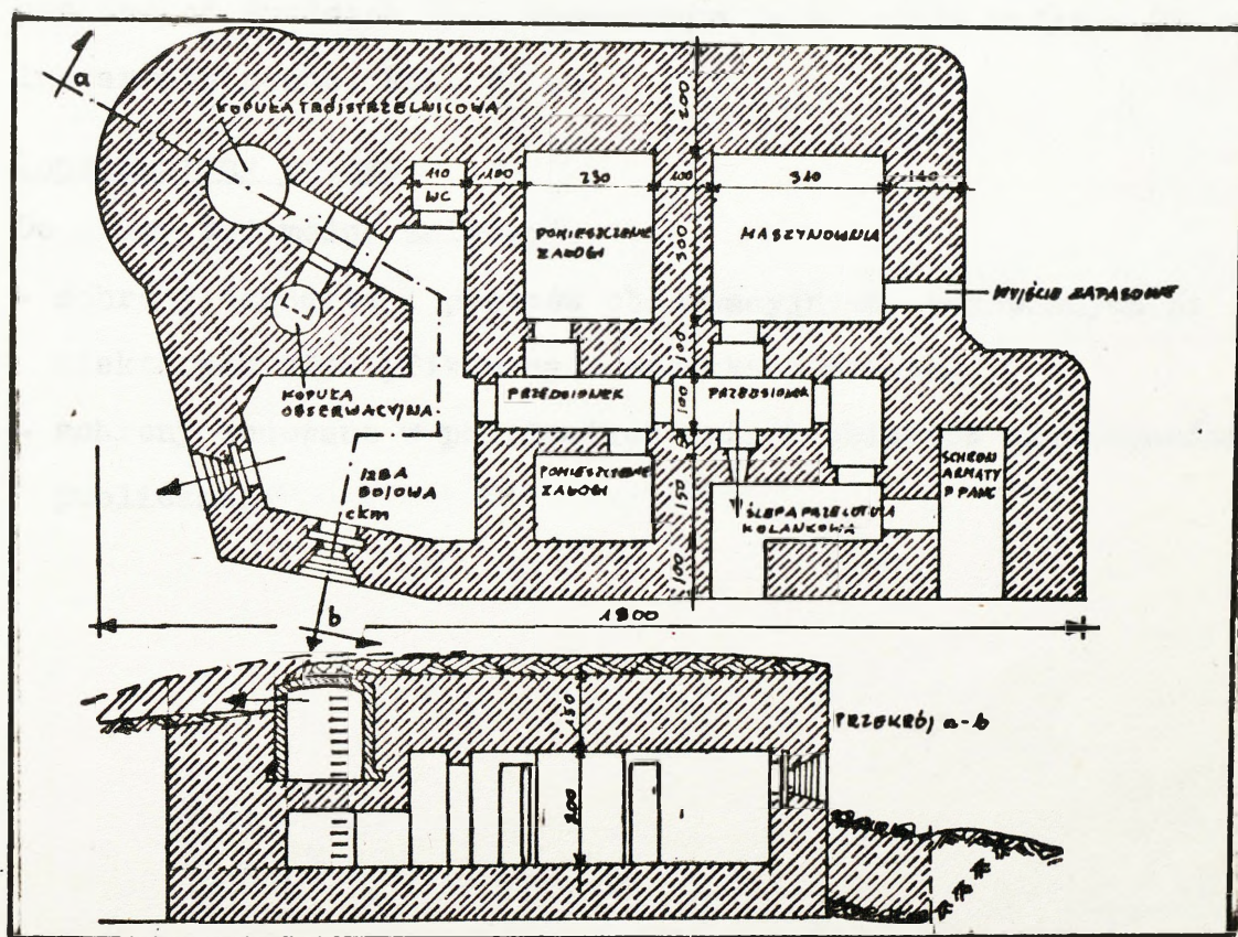
Schron bojowej średniej wielkości
