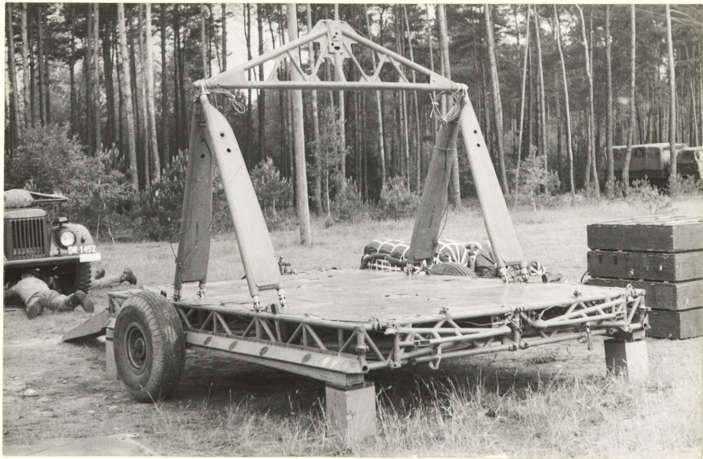
4 PLATFORMA P-127 PRZED ZAŁADOWANIEM SPRZĘTU
