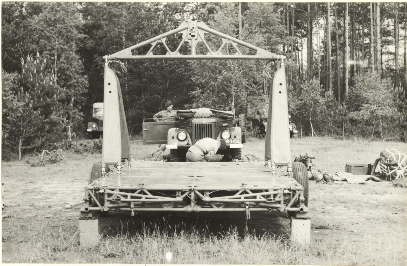
5 SPRAWDZENIE SAMOCHODU GAZ-69 PRZED ZAŁADOWANIEM NA PLATFORMĘ P-127
