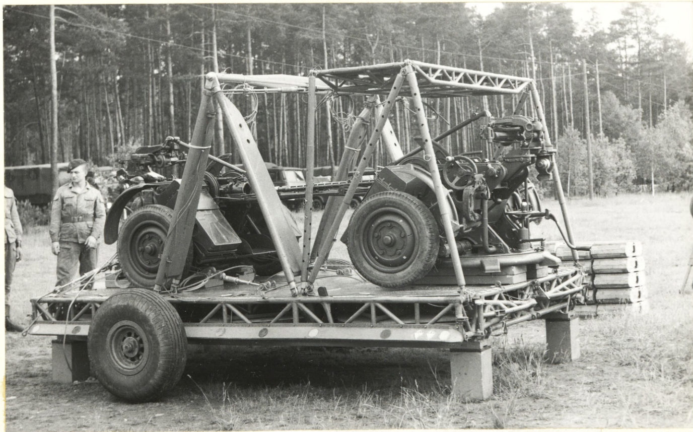
8 PKM-2 ZAŁADOWANE NA PLATFORMĘ P-127
