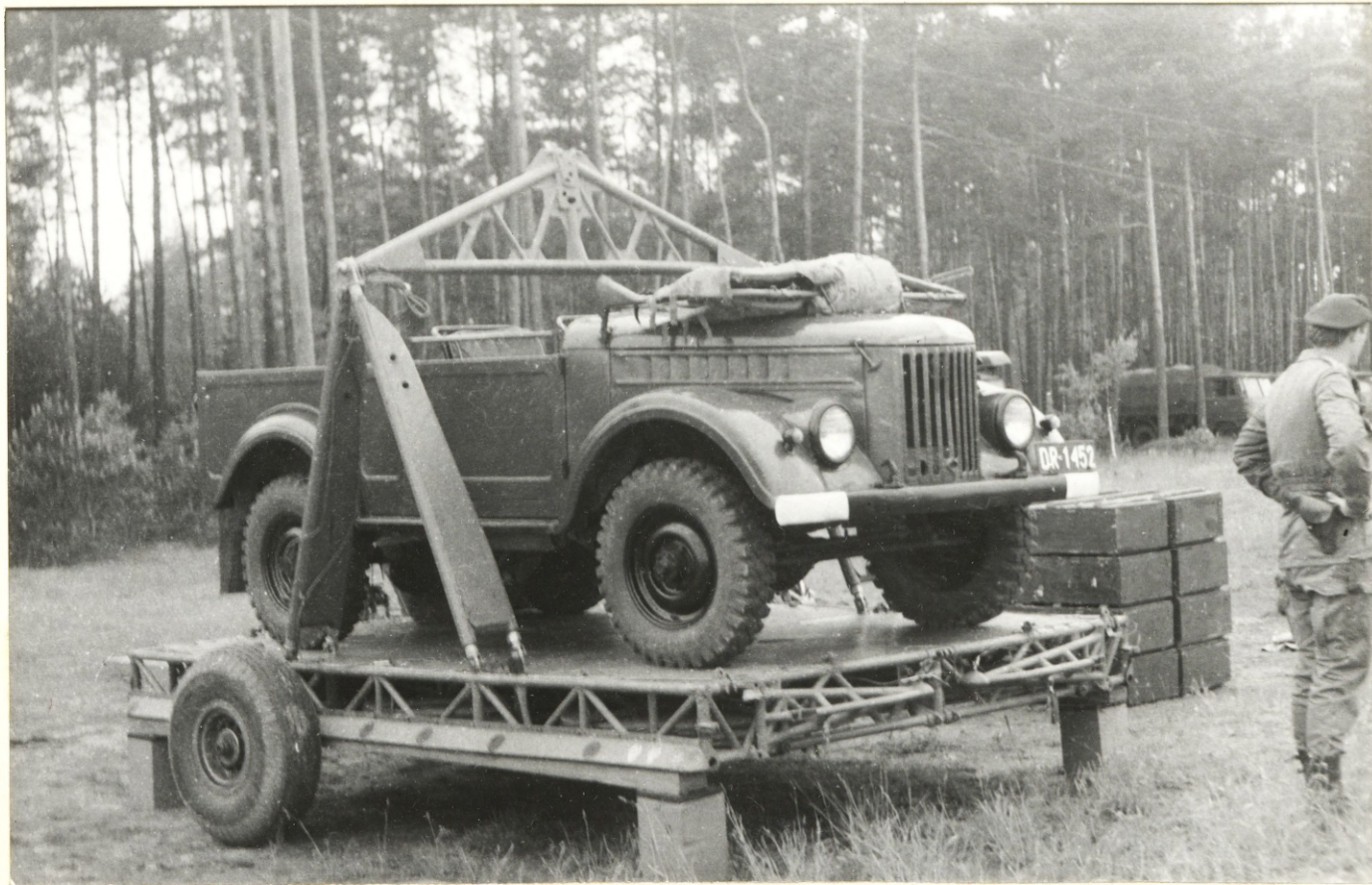
6 SAMOCHÓD GAZ-69 PO WJEŹDZIE NA PLATFORMĘ P-127
