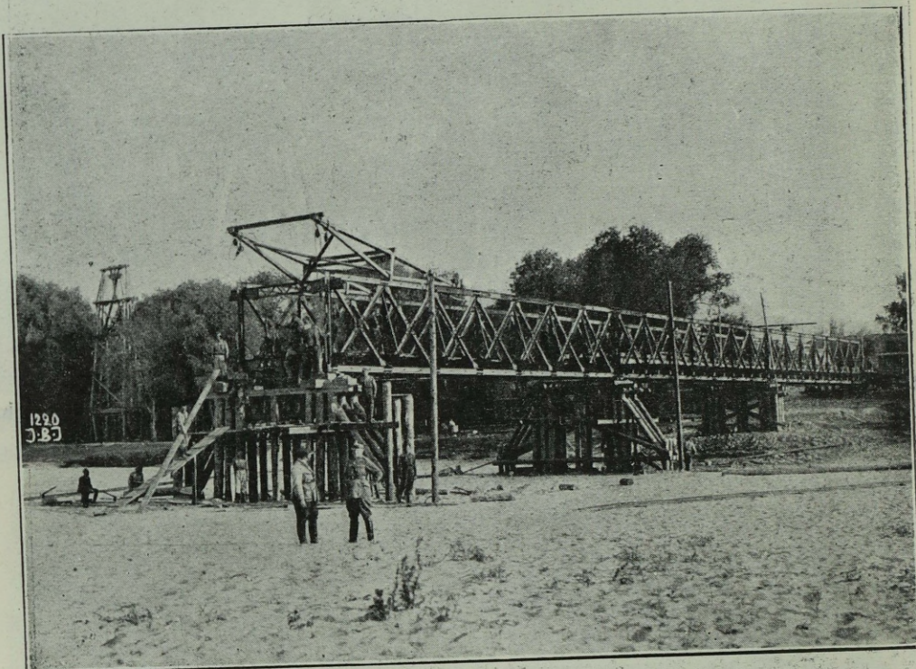
Fot. G 1 . Żelazny, składany most drogowy, jednościenny.
