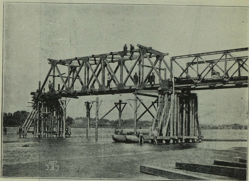
Fot. G 3 . Drewniany składany most drogowy systemu Dworakowskiego (łączenie części drewnianych zapomocą płyt żelaznych i śrub).
