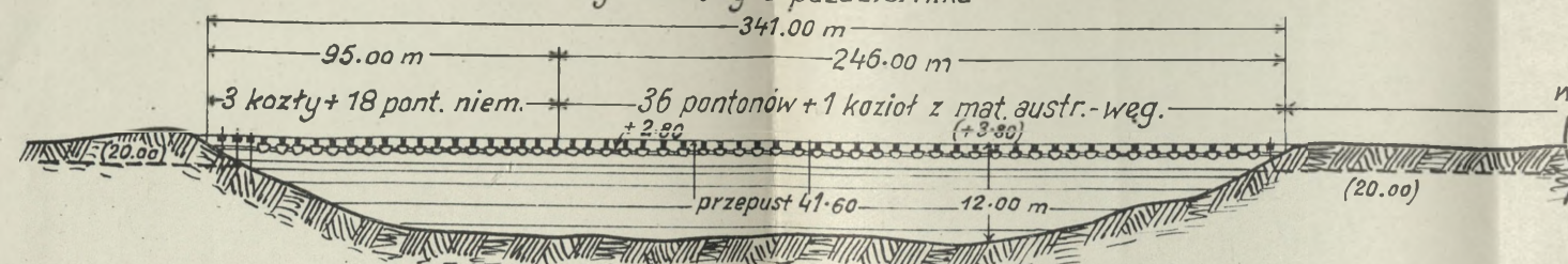
Pierwszy most przez główne ramie pod wyspą Cygańską wybudowany 9 października
