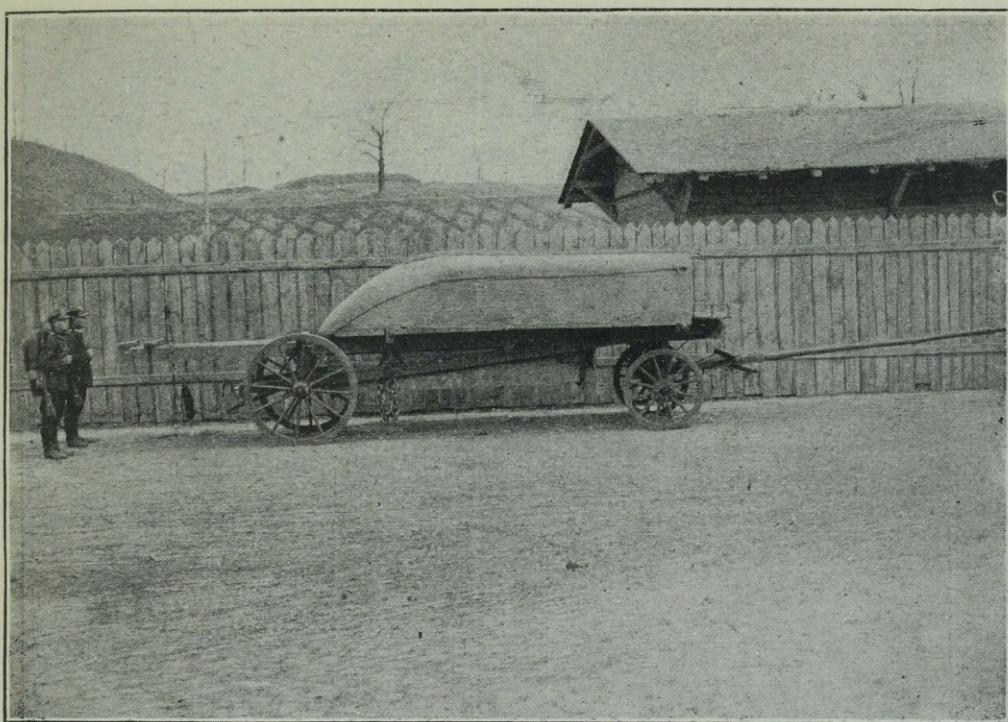
Fot. A 1 . Wóz belkowy kolumny pontonowej.
