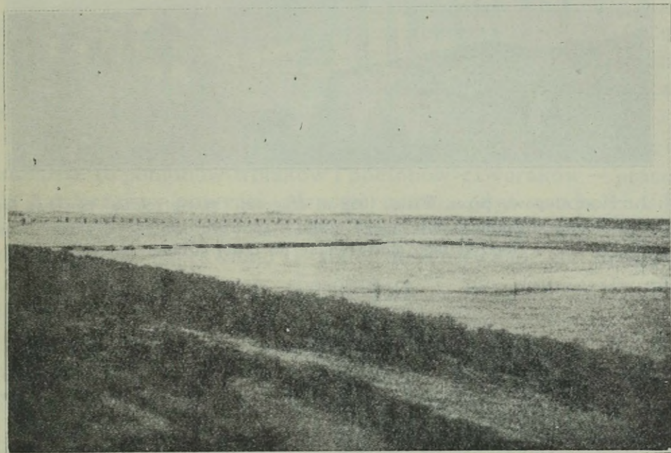
Fot. 2. Most wojenny pod m. Świeże Górne (most nr. 2). Przez piaski na prawym brzegu ułożono dylinę. Na przednim planie widać zagrodę przeciwmینową; z tyłu resztki spalonego mostu rosyjskiego, na których zbudowano most etapowy. Wisła przy niskim stanie wody. Później przedłużono z powodu powodzi most wojenny przez całe koryto rzeki do długości 966 m.
