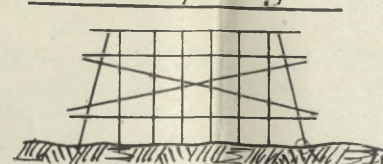
Jarzmo podwójne
