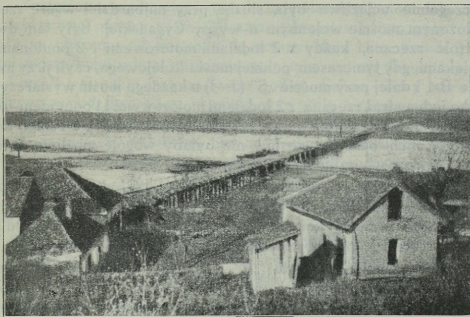
Fot. 11. Austriacko-węgierski most etapowy (część prawa) przez Sawę pod wyspą Cygańską. Całkowita długość mostu 1909 m.
