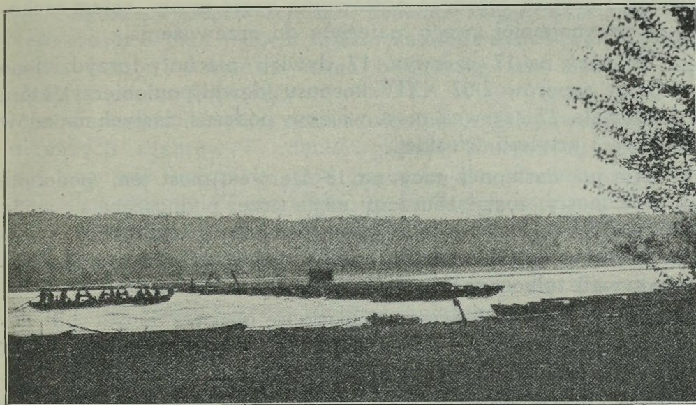
Fot. 17. Most pontonowy 17 dywizji piechoty pod m. C. Mercadelli. Część mostu była w dzień rozrzucona wzdłuż brzegu z obawy przed natarciem lotnictwa nieprzyjacielskiego. Fotografia pokazuje, jak znaczną zmianę w wyglądzie rzeki spowodowała wielka woda w porównaniu z fot. 14 i 15.
