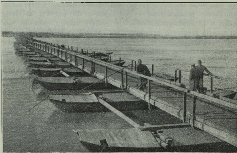
Fot. 8a. Most B-1 z materiału „P”, 365 m długości, wybudowany w ciągu 4½ godzin. (Fotografia mjr. Bisztygi, ówczesnego uczestnika budowy tego mostu. Ze względu na fale podczas silnego wiatru, pontony pokryto deskami). (Przyp. tłum.).
