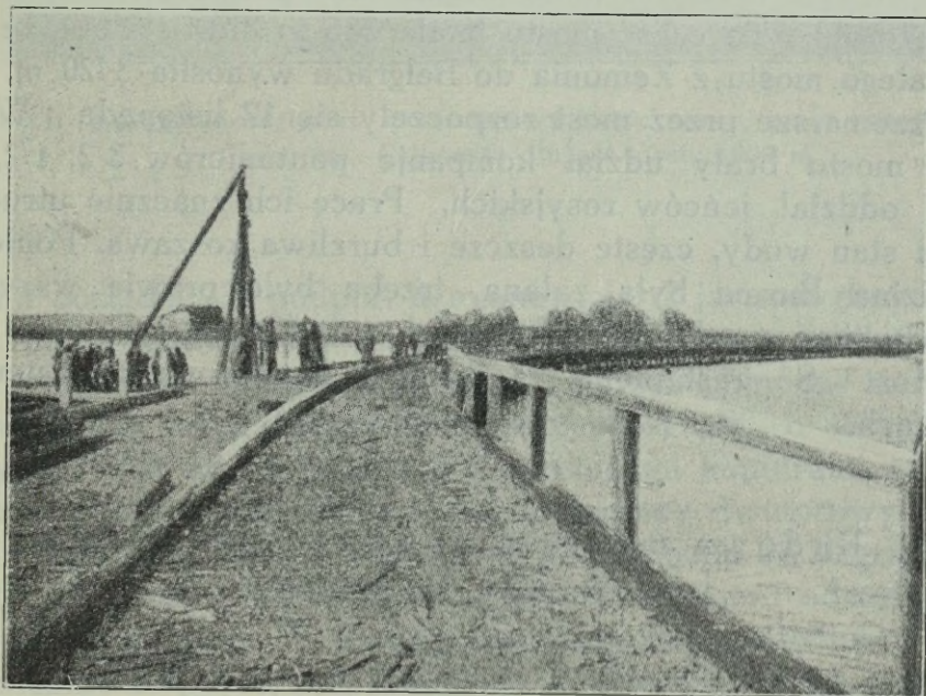
Fot. 10. Austriacko-węgierski most etapowy przez teren zalewowy pomiędzy dworcem kolejowym w Zemuniu a mostem pontonowym przez Sawę koło dworca kolejowego w Belgradzie. Całkowita długość mostu 3420 m.
