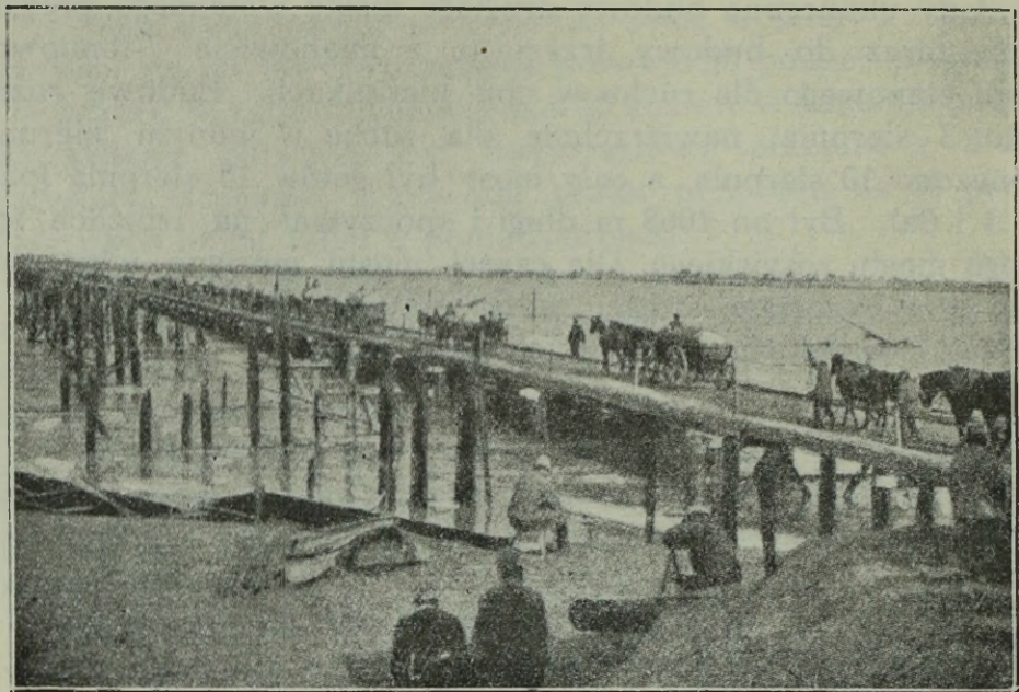
Fot. 3. Most etapowy przez Wisłę, 1068 m długości; nawierzchnia mostowa spoczywa na izbicach dawnego rosyjskiego mostu etapowego, spalonego przez Rosjan. Resztki tego mostu widać po lewej stronie.
