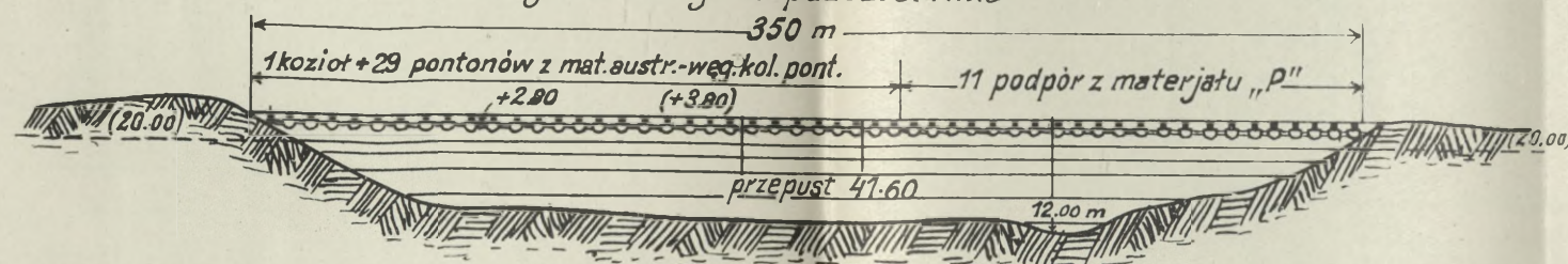
Drugi most przez główne ramie pod wyspą Cygańską wybudowany 14 października
