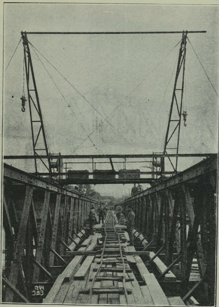
Fot. G 2 . Żelazny, składany most drogowy, dwuścienny; w budowie (jednotorowy).
