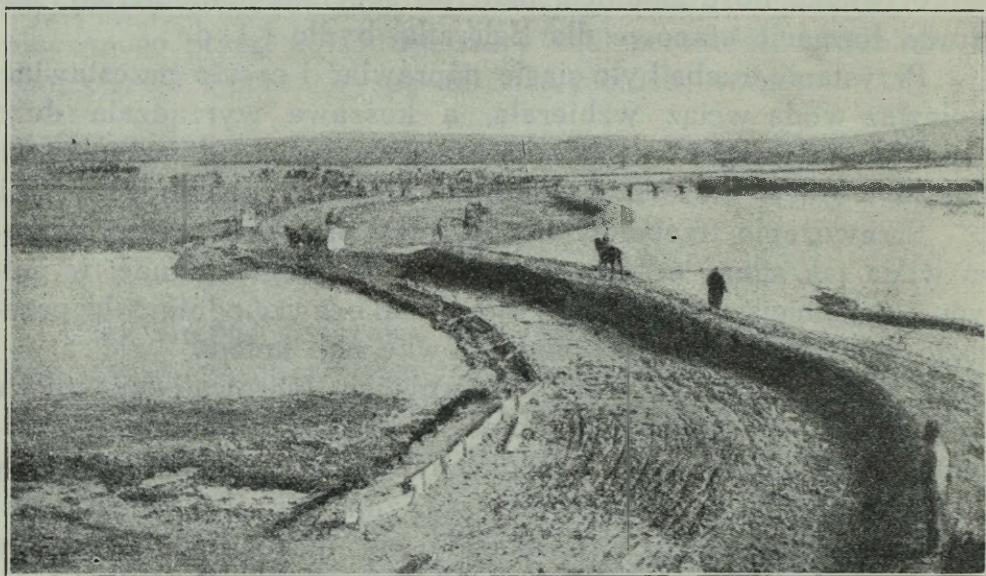
Fot. 9. Most wojenny niemieckiego XXII korpusu rezerwowego przez lewe ramię Sawy pod wyspą Cygańską i dojazd do mostu na lewym brzegu. Most ten wybudowano częściowo (1/3) z niemieckiego częściowo (2/3) z austriackiego materiału przez przynależnych pionierów (pontonierów). Na lewo od mostu stoi przewóz parowy. Z przodu improwizowana grobla przeciw powodzi.
