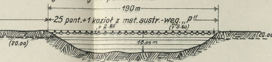
Most „P” - przez ramie południowe wybudowany 10 października
