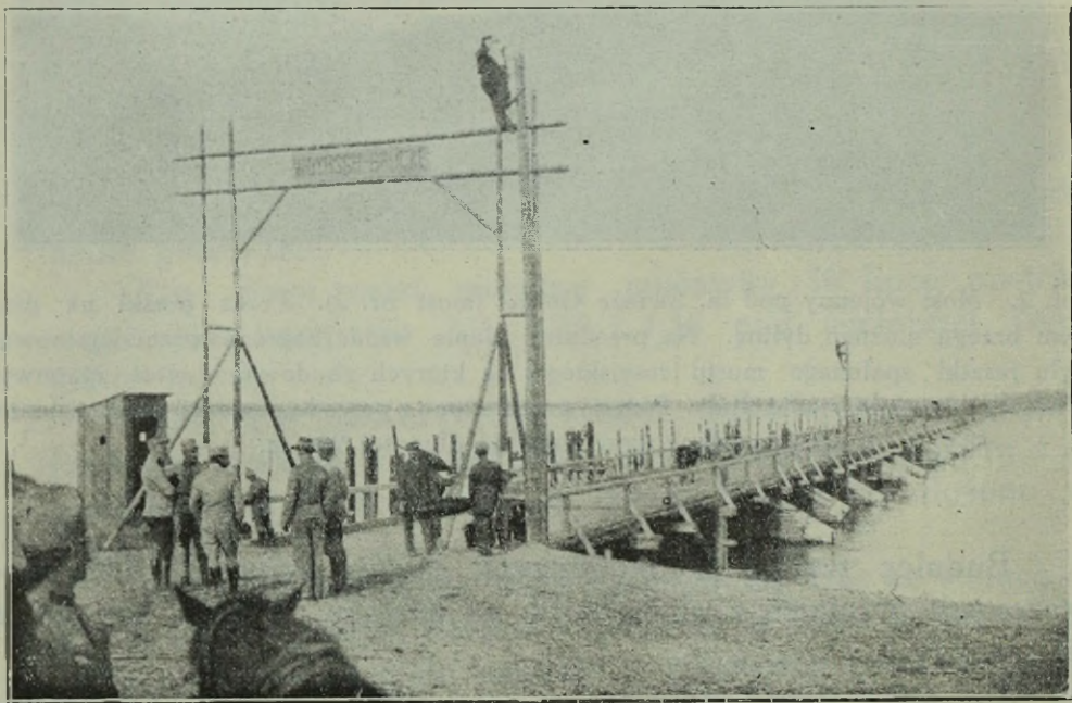
Fot. 3a. Ten sam most etapowy przez Wisłę (jak fot. 3), widziany z góry rzeki. Fotografia dostarczona przez mjr. saperów Bisztygę, ówczesnego uczestnika przeprawy (przyp. tłum.).
