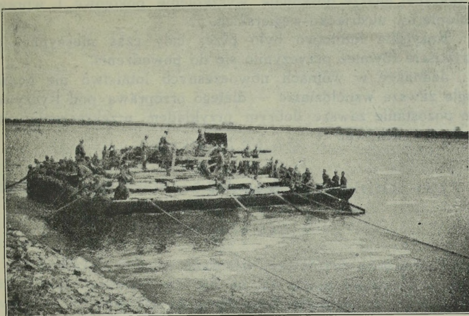
Fot. 4. Przewożenie dział 15 cm niemieckiego, 15 tonnowego, przez pontonierów austriackich. Człon z 4 pontonów-czworaków, holowany w górę rzeki (na lewym brzegu) przy pomocy dwóch pontonów-czworaków, przyczepionych do boków członu.
