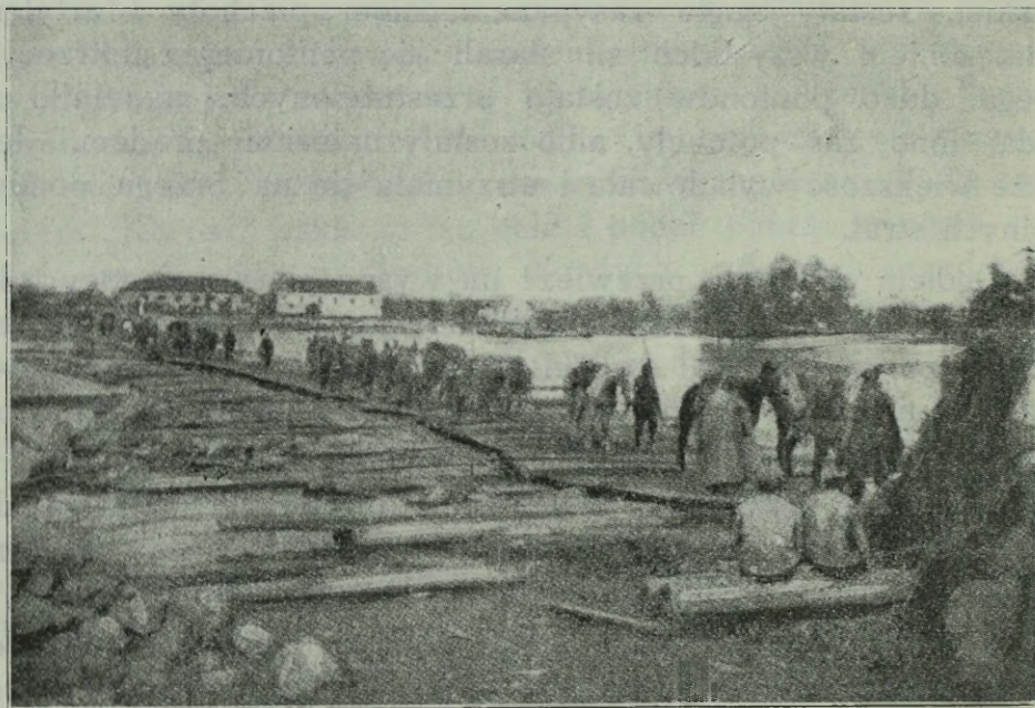
Fot. 8. Serbski most tratwowy przez prawe ramię Sawy pod wyspą Cygańską. Po zdobyciu wyspy Cygańskiej piechota niemiecka natarła przez ten most na prawy brzeg Sawy.
