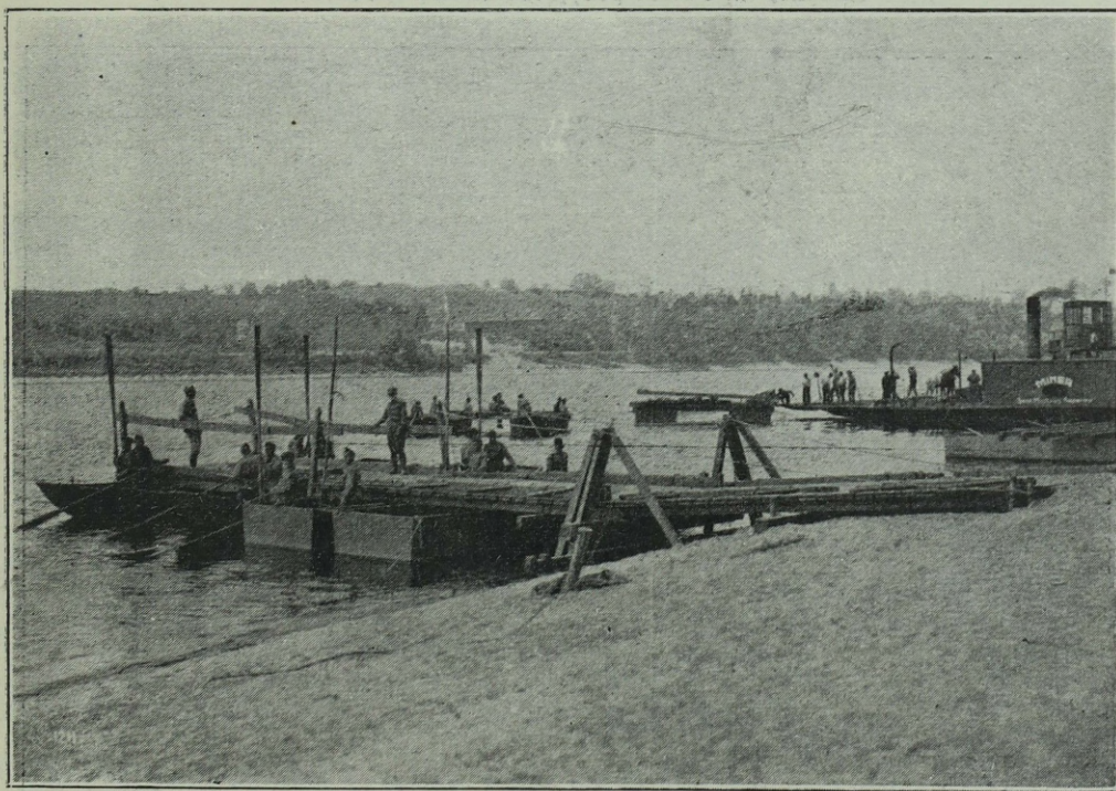
Fot. D 3 . Lekki człon koło wzmocnionej przystani. Powyżej przewóz parowy „Miner”.
