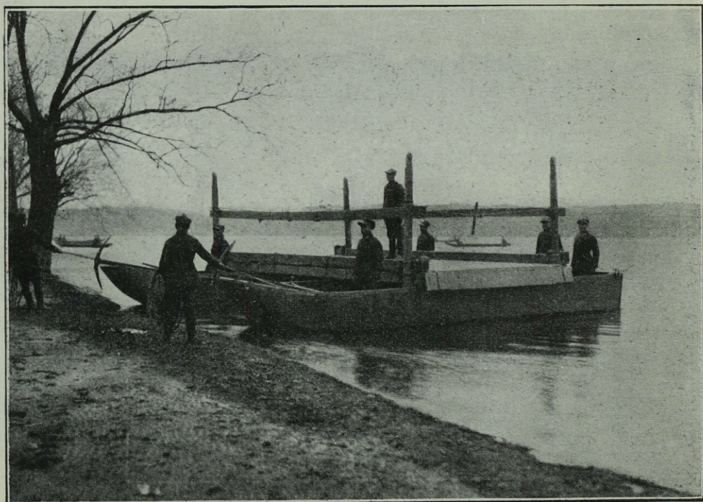
Fot. D 1 . Lekki człon przewozowy na 60 ludzi po wylądowaniu.
