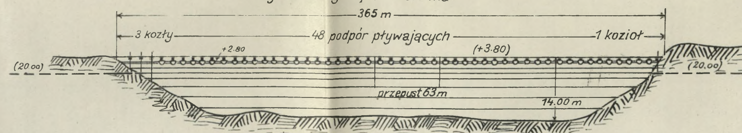
Ciężki dwutorowy most etapowy pomiędzy dworcem kol. m. Zemun a Belgradem - Jarzma takie same jak powyżej
