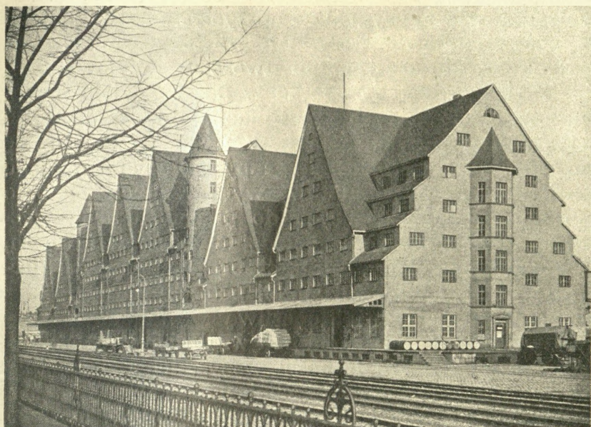
SKŁADY TOWAROWE W KOLONII NAD RENEM — PRZYKŁAD WSPÓŁCZESNEJ ARCHITEKTURY UŻYTKOWEJ O SWOISTEM PIĘKNIE
