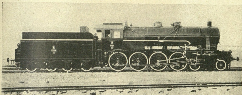
PAROWÓZ OSOBOWY, UŻYWANY W P. K. P. DO POCIĄGÓW POSPIESZNYCH — KAŻDA FORMA WYNIKA Z WŁAŚCIWOŚCI MATERJAŁU I FUNKCYJ, KTÓRE SPEŁNIA
