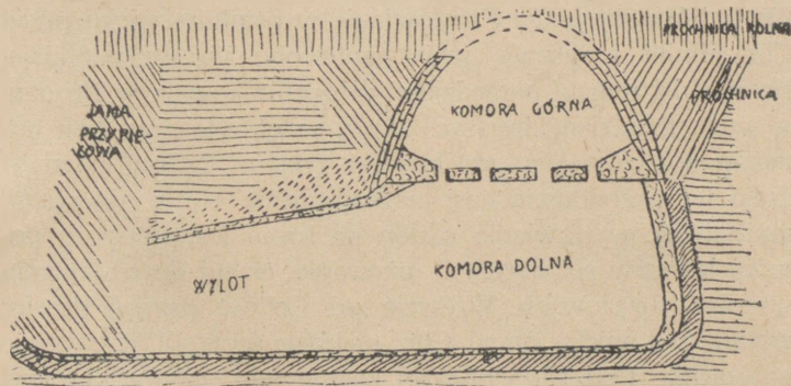
Ryc. 63. Piec garncarski z młodszego okresu rzymskiego z Tropiszowa, w pow. miechowskim (w przekroju podłużnym).
