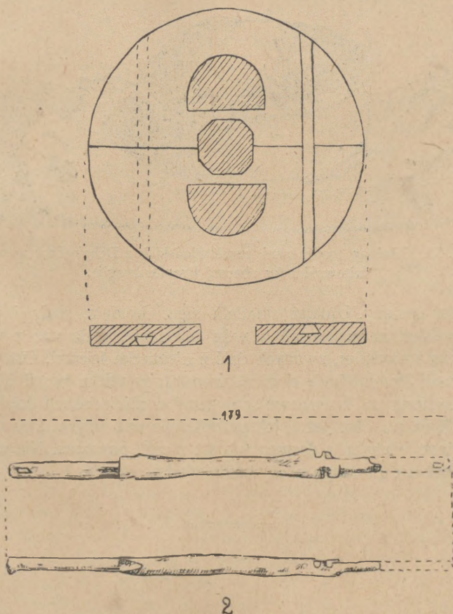
Ryc. 50. Koło tarczowate i oś wozu prasłowiańskiego z Biskupina.
