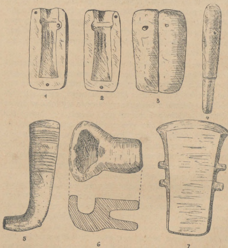
Ryc. 34. Formy odlewnicze ze Śląska (1—4), 5. gliniany koniec miecha kowalskiego ze Śląska, 6. gliniany tygiel odlewniczy z Biskupina, 7. kowadło brązowe z Przemyśla.
