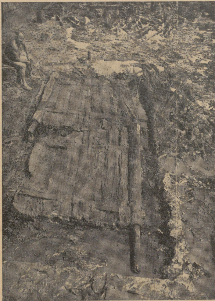
Ryc. 38. Wrota grodu biskupińskiego. Obie połowy leżą tu ponad sobą, nie obok siebie.
