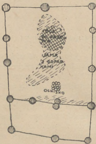
Ryc. 13. Prasłowiański dom słupowy z Tarnowy, w pow. konińskim (dawniej słupeckim) z wczesnego okresu żelaznego (700 - 400 przed Chr.).
