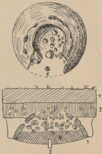
Ryc. 65. Piec hutniczy z I wieku po Chr. z Mechlina, w pow. śremskim.
