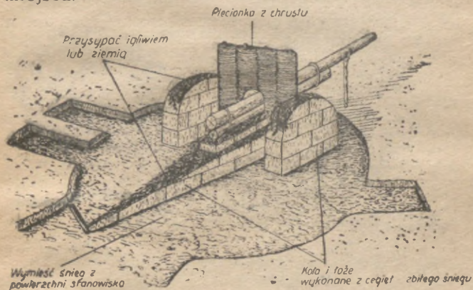
Rys. 37. Pozorna, 76 mm armata wykonana w warunkach zimowych. Czas budowy: 4 żołnierzy, 2 godziny
