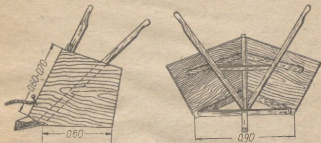
Rys. 26. Pług drewniany do budowy rowów pozornych w śniegu. Czas budowy 10 mb. rowu za pomocą pługa; 6 strzelców, 5—7 minut
