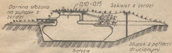
Rys. 41. Maskowanie czołga umieszczonego w okopie. Czas maskowania przez załogę — 3,5 godziny
