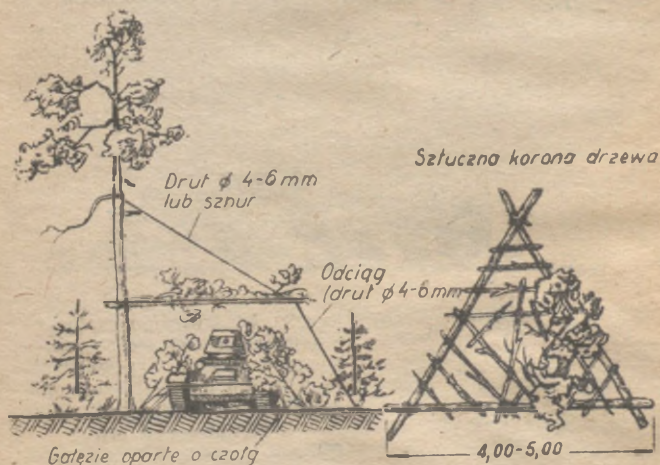
Rys. 40. Sztuczna korona drzewa. Czas budowy jednej korony: 3 żołnierzy, 1 godzina
