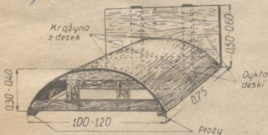
Rys. 21. Przenośne szalowanie do budowy sklepienia ze śniegu
