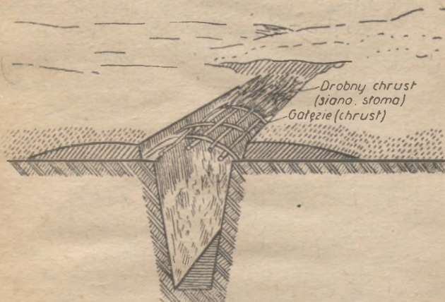
Rys. 19. Maskowanie rowu przykryciem wypukłym. Czas maskowania 10 mb: dwóch strzelców 2 godziny
