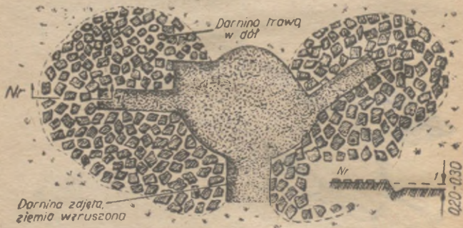
Rys. 38. Pozorne stanowisko artyleryjskie. Czas budowy: 3 żołnierzy, 1,5 godziny
