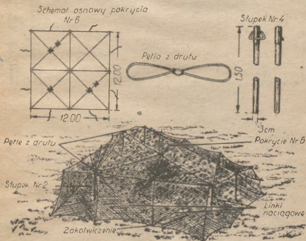
Rys. 27. Maska typu „A” dla dział pułkowego. Komplet maski: pokrycie nr 6 — 1 szt.; słupek nr 2 — 5 szt.; siatka nr 4 — 1 szt.; pętla z drutu — 15 szt., pokrowiec zwijany nr 6 — 1 szt. Czas maskowania działła przez obsługę — 20 minut
