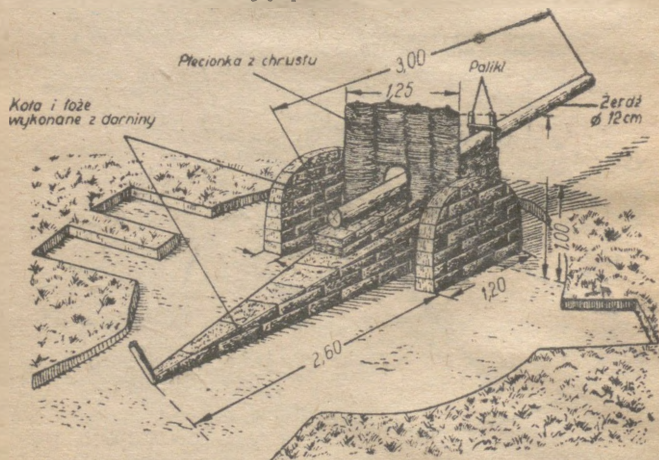
Rys. 36. Pozorna 76 mm armata wykonana w warunkach letnich. Czas budowy: 5 żołnierzy, 1,5 godziny
