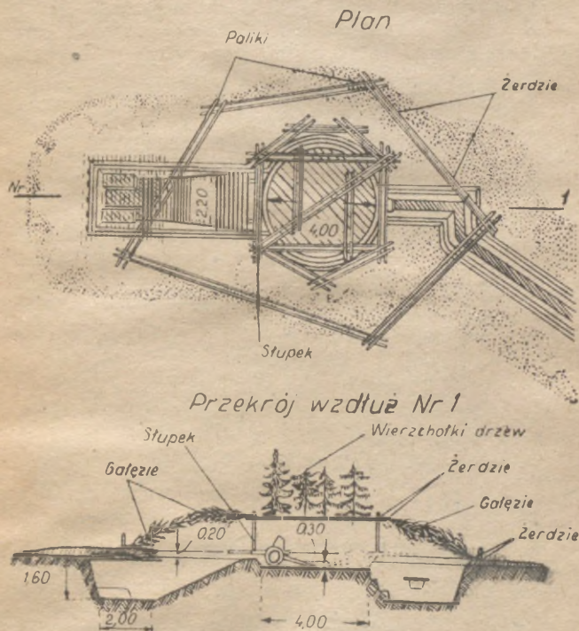
Rys. 33. Maskowanie działa przeciwpancernego pod grupą krzaków. Czas maskowania przez obsługę działa — 3 godziny
