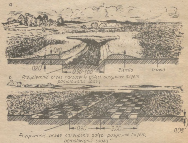
Rys. 25. Budowa rowu pozornego: a) kopanie rowu o niepełnej głębokości. Czas budowy 10 mb.: 1 strzelec 2 godz. 30 minut.; b) zdjęcie darniny. Czas budowy 10 mb.: 1 strzelec 4 godziny. Zdjętą darninę można wykorzystać do maskowania rowów rzeczywistych
