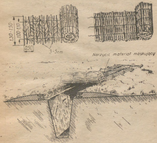
Rys. 15. Budowa i zastosowanie mat ze słomy i chrustu. Czas przygotowania 10 mb: 3 rob.-godzin
