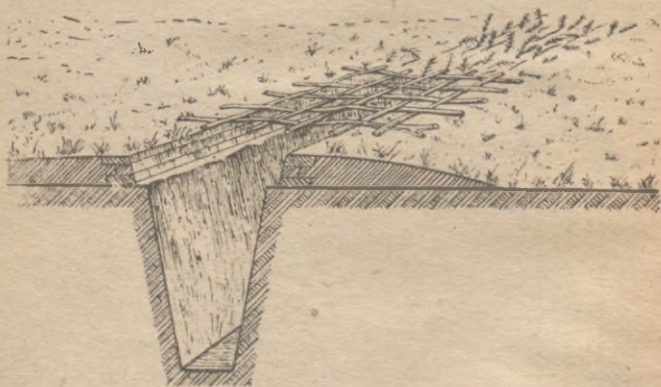
Rys. 14. Budowa i zastosowanie plecionek z chrustu. Czas przygotowania jednej plecionki: 0,5 rob.-godzin
