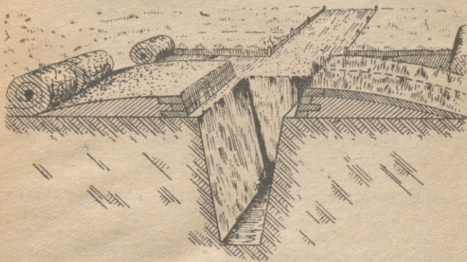
Rys. 11. Sposób maskowania przedpiersia pasami darniny
