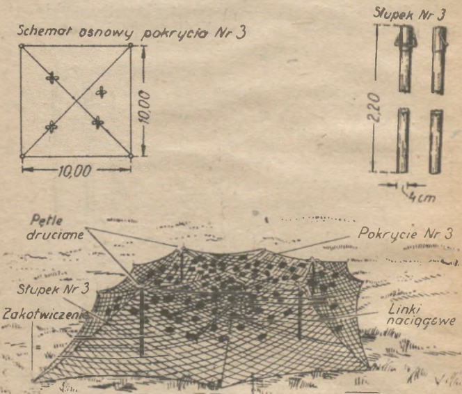
Rys. 28. Maska typu „E” dla dział przeciwpancernego. Komplet maski: pokrycie nr 3 — 1 szt.; słupki nr 3 — 4 szt.; siatka nr 4 — 1 szt.; pętla druciana — 12 szt.; pokrowiec zwijany — 1 szt. Czas maskowania dział przez obsługę — 15 minut
