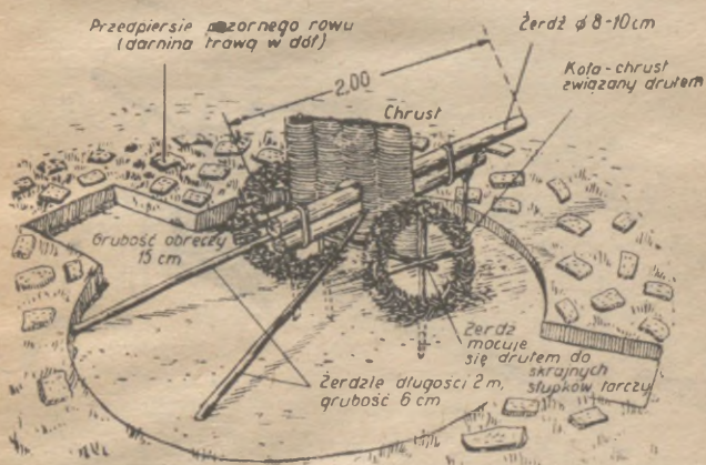
Rys. 35. Pozorna armata przeciwpancerna. Czas budowy przez 3 strzelców — 2 godziny
