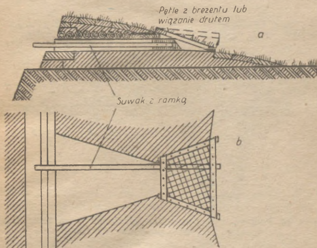
Rys. 13. Budowa ramki ruchomej przed strzelnicą
