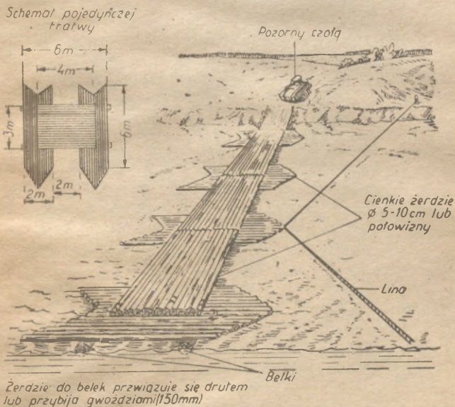
Rys. 48. Pozorny most na podporach pływających z żerdzi
