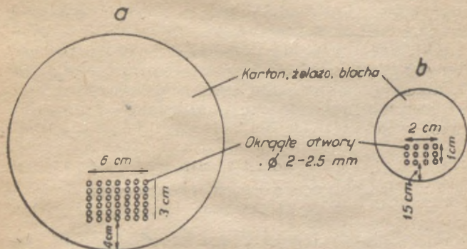
Rys. 44. Tarcza zaciemniająca: a — dla latarni; b — dla sygnałów „stop”
