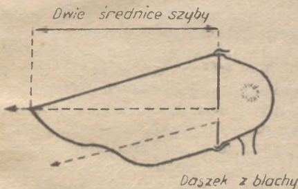
Rys. 45. Latarnia lub sygnał „stop” z umieszczonym daszkiem z blachy
