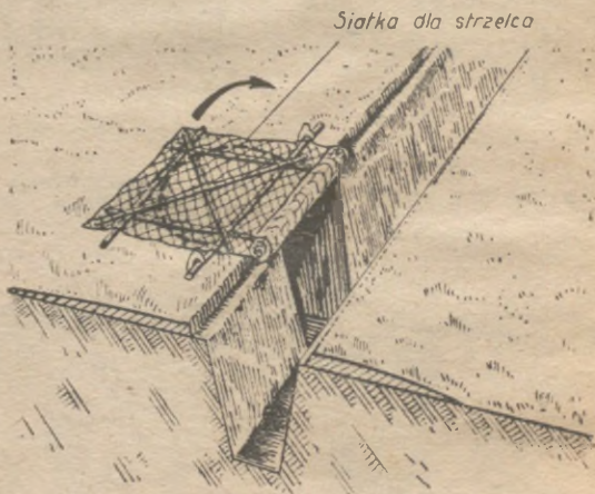
Rys. 16. Maskowanie stanowiska strzeleckiego siatką dla strzelca. Czas budowy: 1 strzelec 10—15 minut
