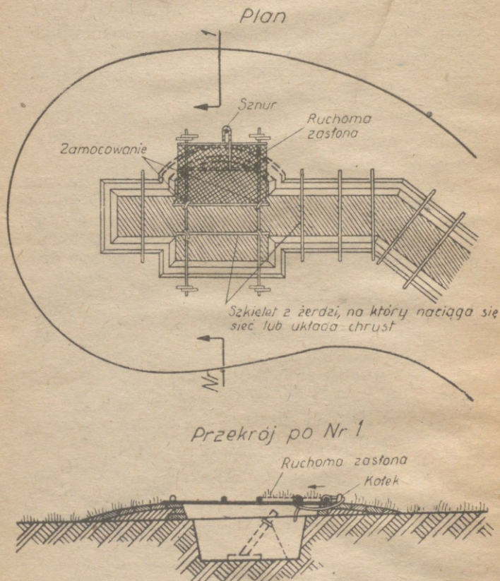
Rys. 34. Maskowanie stanowiska moździerza. Konstrukcja szkieletu i zastony ruchomej. Czas maskowania przez obsługę — 45 minut
