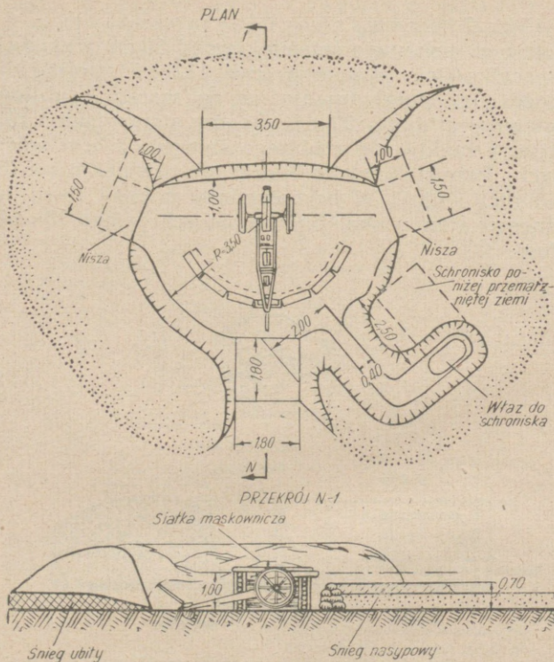
Rys. 113. Stanowisko 76 mm działu pułkowego
