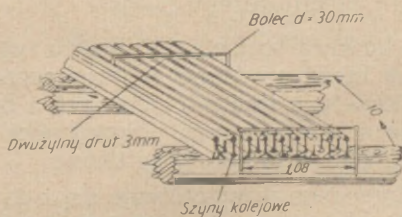
Rys. 156-b. Warstwa detonacyjna z szyn
