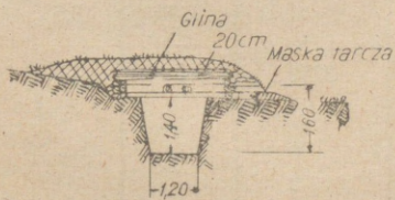
Rys. 44. Stanowisko obserwacyjne dowódcy (typ lekki)
