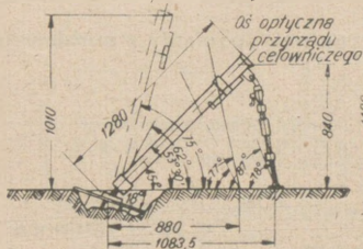
92mm móżdziej batalionowy wzoru 1938 (położenie bojowe)
