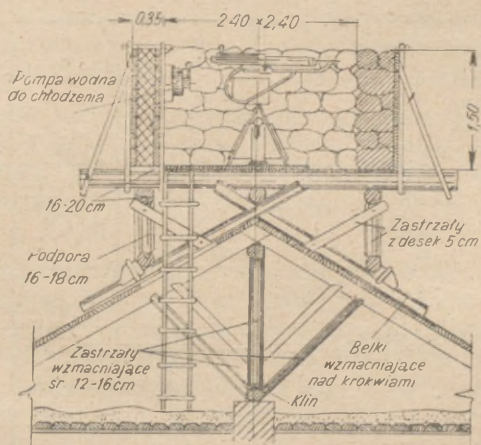
Rys. 91 Stanowisko na dachu dla czterech sprzężonych ckm przeciwlotniczych
