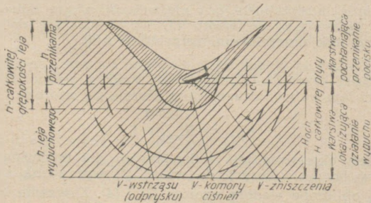
Rys. 3. Schemat burzącego działania pocisku (bomby lotniczej) w warstwie ochronnej
