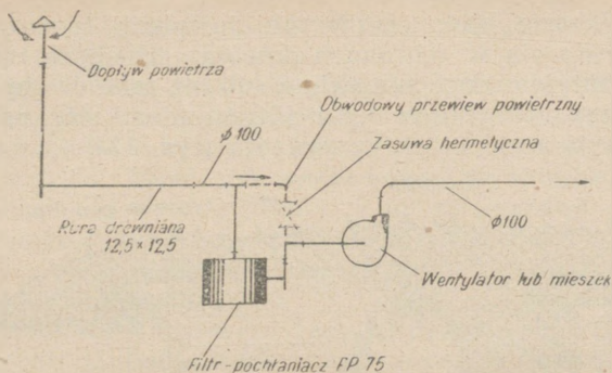
Rys. 135. Schemat instalacji FP-75 z wentylatorem (wymiary: rury drewnianej w cm, przewodu powietrznego w mm)
