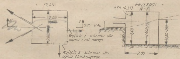
Rys. 5. Schemat schronu dla ckm
