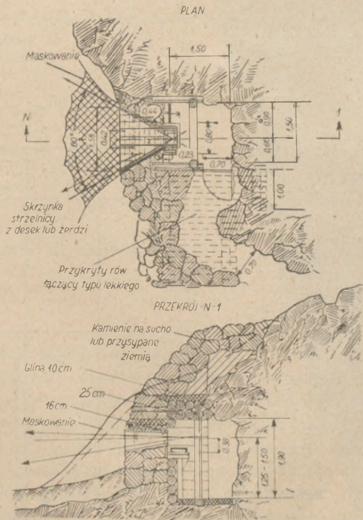
Rys. 104. Wzmocniony lub ciężki schron dla ckm na wpeł wglębiony w pieczarę
