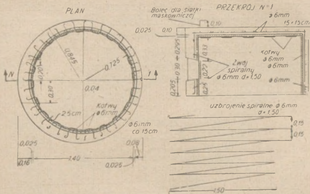
Rys. 160. Kopuła żelazobetonowa
