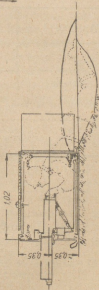
Rys. 17. Składana kopuła pancerna dla ckm typu MNTP przeciw odłamkom; ustawienie I — dla strzelania w pozycji leżącej. Ustawienie II — dla strzelania stojąc
