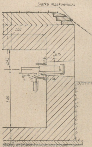
Rys. 120. Umocowanie ckm na półce w schronie żelazobetonowym
