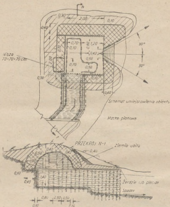
Rys. 7. Stanowisko dla ckm ze stropem wiklinowym
