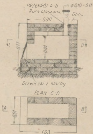
Rys. 139. Najprostrzy piec z cegiel
