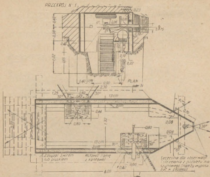
Rys. 19. Wykorzystanie kadłuba przewróconego czołga jako ostrogu dla ckm
