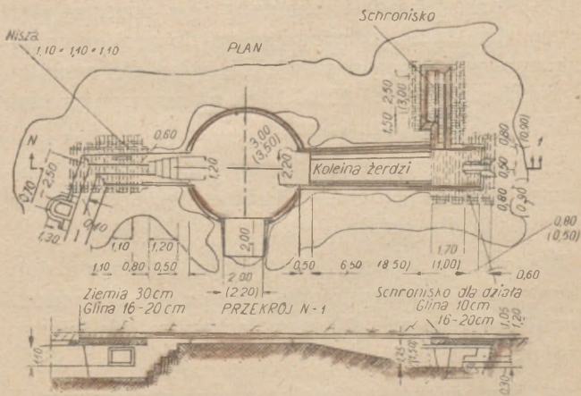
Rys. 37. Stanowisko dla 45 mm dział przeciwzołgowego oraz dla 76 mm dział artylerii pułkowej (wymiary podane w nawiasach odnoszą się do dział 76 mm)
