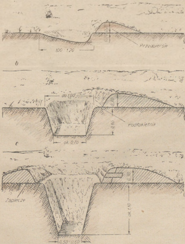
Rys. 3. Doły strzeleckie: a) dla strzelania leżąc (wnęć strzelecki); b) dla strzelania w postawie klęczącej; c) dla strzelania w postawie stojącej.
