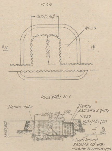
Rys. 97. Stanowisko ziemne dla moździerza w terenie leśno-bagiennym. Wymiary są podane dla moździerza 120 mm, w nawiasach dla moździerza 82 mm
