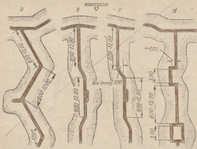
Rys. 57. Narysy rowów łączących: a) zygzakami; b) łamanymi; c) schodami; d) z poprzecznicami
