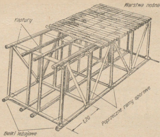
Rys. 153. Szkielet konstrukcji jężmowej wzmocnionej ramami poprzecznymi
