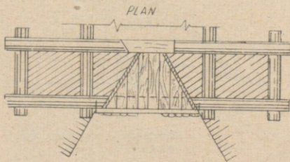
Rys. 124. Maskowanie strzelnicy zasłoną rozsuwaną
