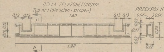
Rys. 161. Prostokątna belka żelazobetonowa
