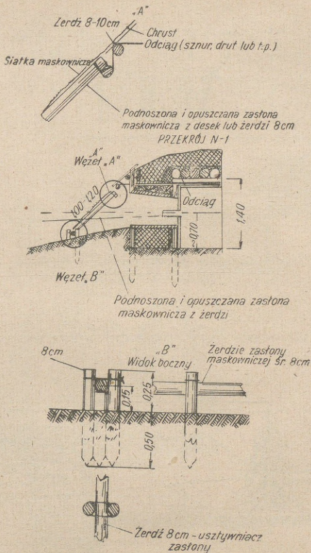
Rys. 123a. Przekrój nr 1 i szczegóły do rys. 123
