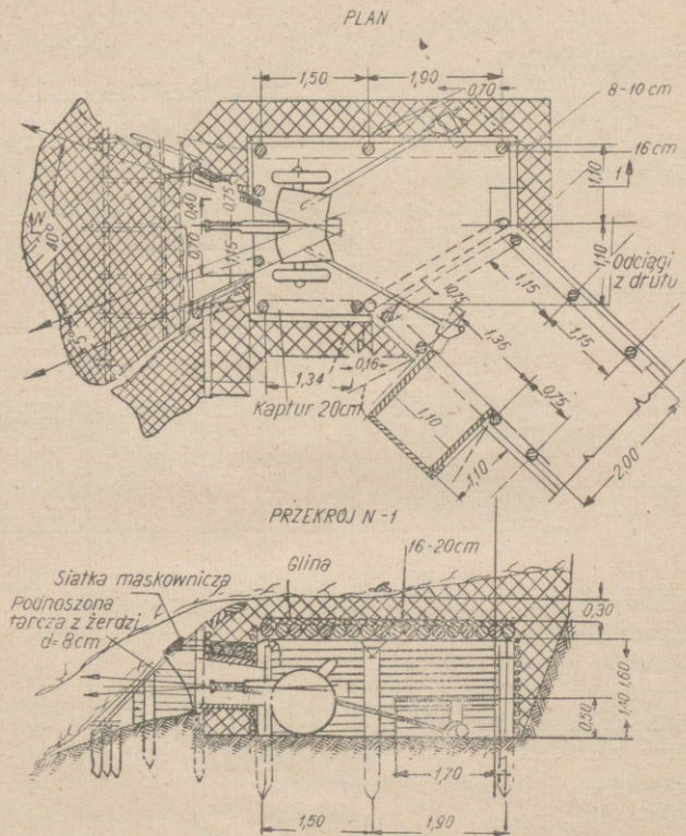
Rys. 40. Lekki bojowy schron drewniany dla działa
