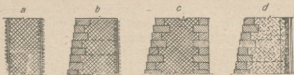
Rys. 143. Typowe odziewanie ścian w konstrukcjach ziemnych: a) odziewanie pleciakami; b) odziewanie pleciakami z darnią; c) odziewanie darnią; d) odziewanie darnią z żerdziami.
