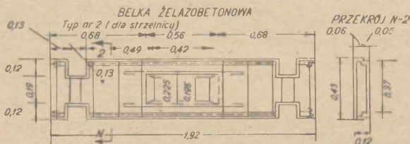
Rys. 162. Belka ze strzelnicą
