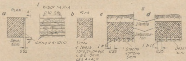
Rys. 169. Szczegóły warstwy przeciwdypryskowej w obiekcie żelazbetonowym:
