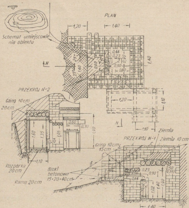
Rys. 28. Składana żelazobetonowa półkaponiera dla ckm, typ wzmocniony
