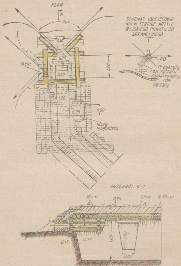
Rys. 41. Lekki drewniany punkt obserwacyjny
