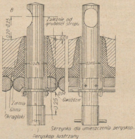
Rys. 125. Ustawienie peryskopów:
