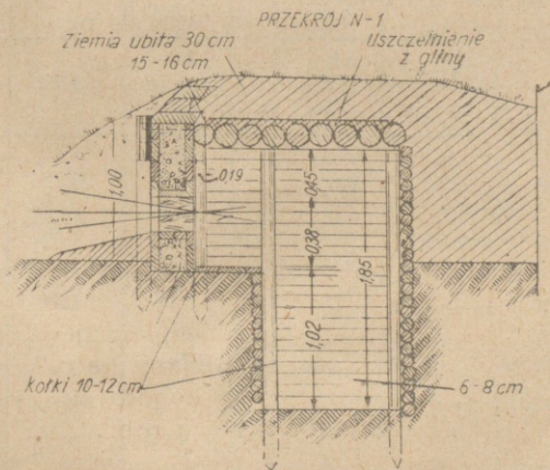
Rys. 12. Łekki schron nasypowy dla ckm (szalówka ścianek z desek)
