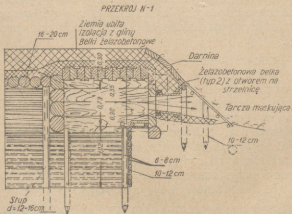
Rys. 15. Żelazobetonowy schron składany, z belek żelazobetonowych i drewnianych
