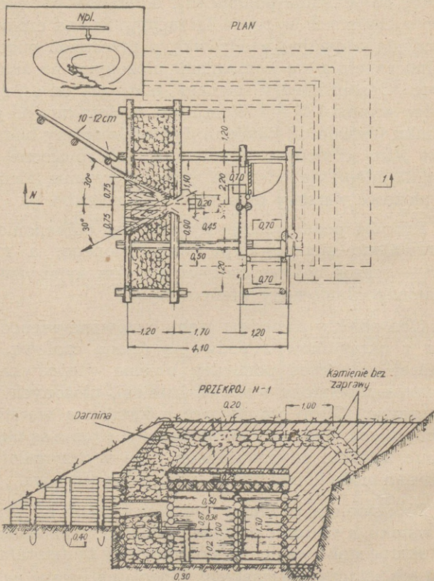
Rys. 24. Drewniana półkaponiera dla ckm, typ wzmocniony
