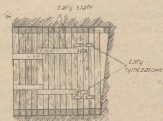
Rys. 176. Pędzenie chodników poziomych w gruntach twardych
