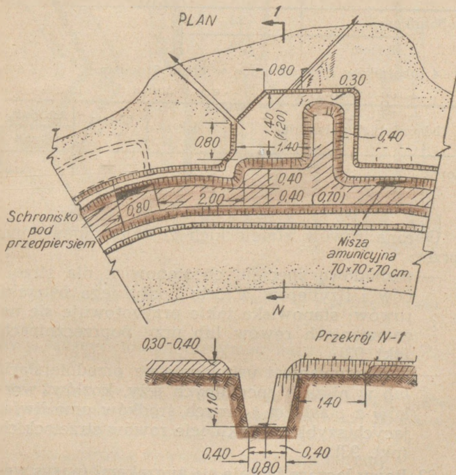
Rys. 56. Stanowisko uniwersalne
