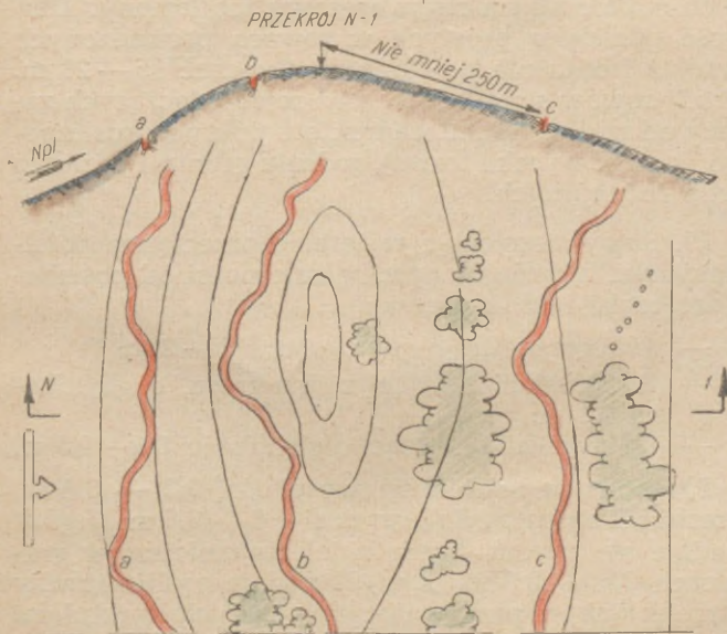
Rys. 52. Umieszczenie ciągłych rowów strzeleckich w terenie: a) na stoku; b) na grzbiecie topograficznym; c) na przeciwstoku
