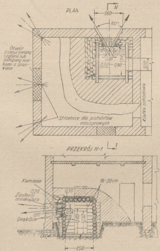
Rys. 37. Wzmocniony schron dla ckm w domu murowanym
