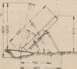
82mm móżdziej batalionowy wzoru 1941 (położenie bojowe)
