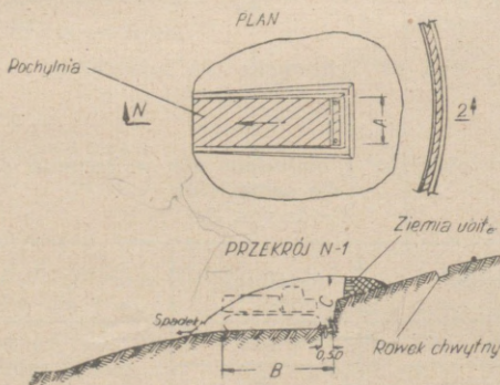
Rys. 85. Schronisko dla traktora
