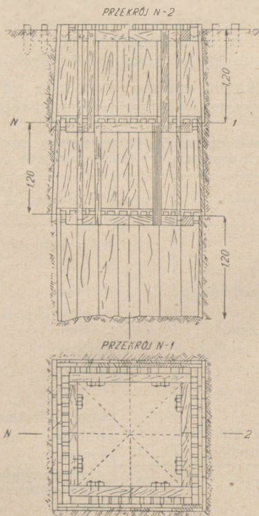
Rys. 181. Zapuszczanie szybu w gruntach lekkich (typ II)
