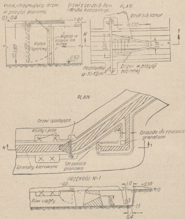
Rys. 68. Urządzenie drzwi opadających i stanowiska strzeleckiego dla obrony wewnętrznej rowu strzeleckiego lub łączącego
