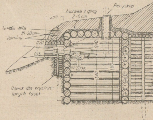
Rys. 119. Umocowanie ckm na półce w schronie drewnianym
