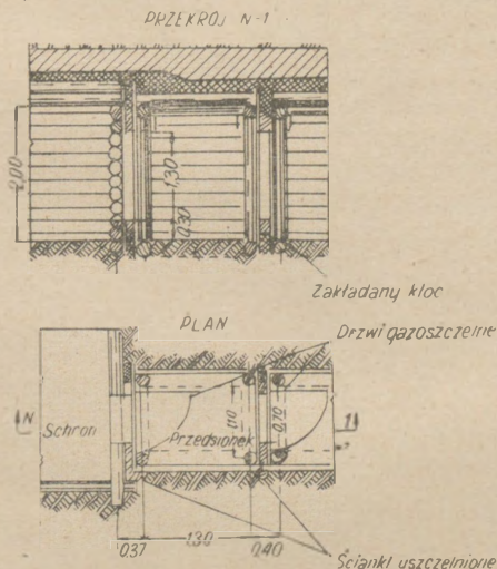
Rys. 127a. Przedsionek z uszczelnionymi przegrodami poziomymi
