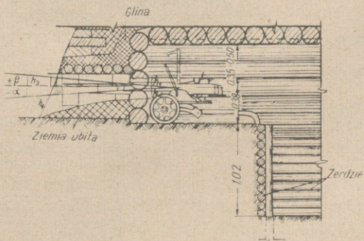
Rys. 115. Umocowanie ckm na nieruchomym stole, ustawienie uchwytu poziome
