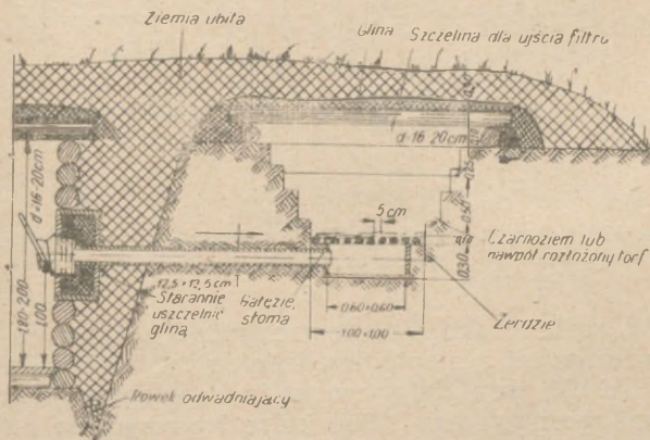
Rys. 134. Instalacja filtru-wentylacyjna z materiałów podręcznych
