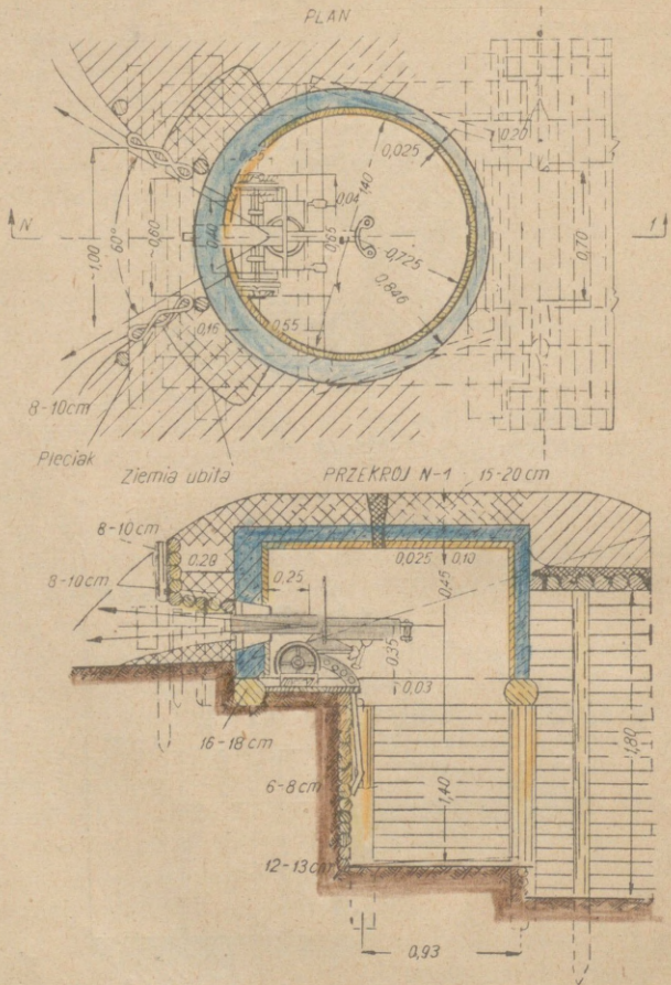
Rys. 14. Żelazobetonowa kopuła dla ckm
