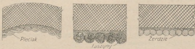
Rys. 144. Typowe stropy w konstrukcjach ziemnych
