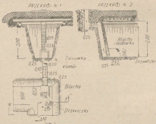
Rys. 140. Piec-kominiek urządony w ziemi
