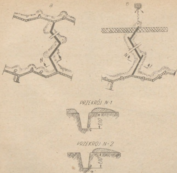
Rys. 70. Kąpanie rowów łączących i strzeleckich systemem sapy; a) z wysypką przedpiersia z jednej strony; b) z wysypką przedpiersia z obu stron
