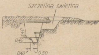
Rys. 44. Stanowisko obserwacyjne dowódcy (typ lekki)
