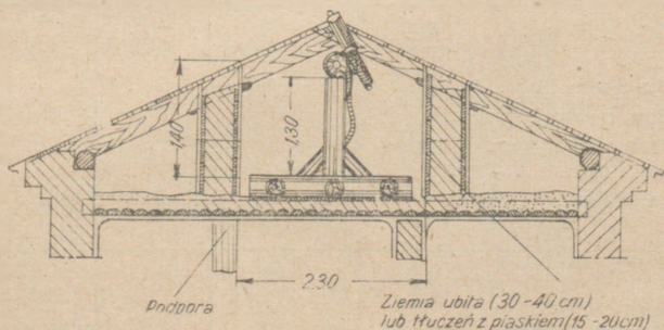
Rys. 90. Stanowisko przeciwlotnicze dla ckm na strychu
