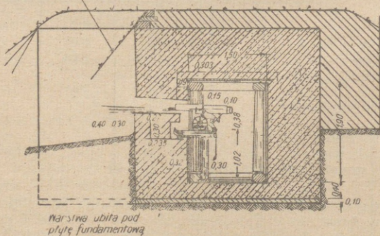
Rys. 30. Monolitowa żelazbetonowa półkaponiera dla ckm (typ ciężki). W przekroju podany przykład szalowania wewnętrznego, pozostającego na stałe w budowni
