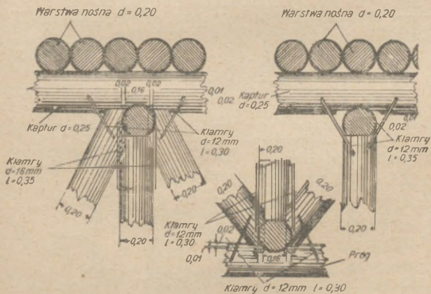
Rys. 153-a. Szczegóły połączeń (do rys. 153)
