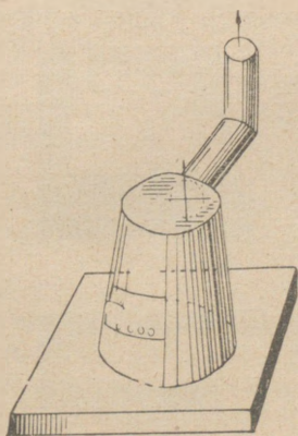
Rys. 138. Piecyk zaimprovizowany z opakowania blaszanego (z wiadra)
