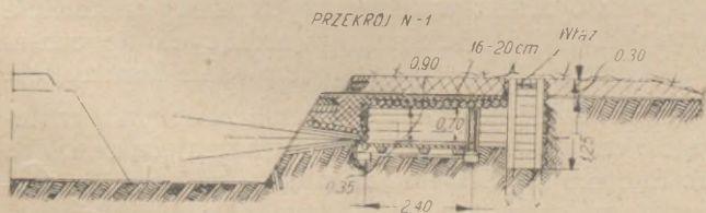
Rys. 11. Lekki schron dla pistoletu maszynowego lub rkm wbudowany w skarpę rowu przeciwczołgowego i przystoso- wany do strzelania leżąc
