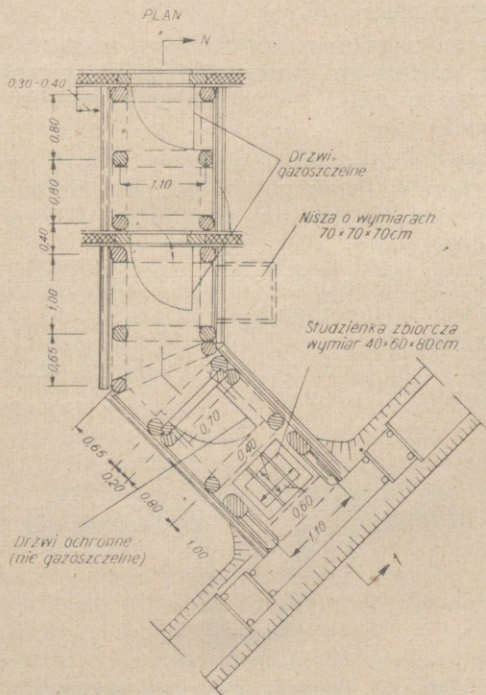
kys. 157. Wejście do schronu drewnianego (drugi przedsionek nie jest uwidoczniiony pkt 174)
