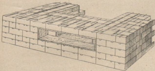
Rys. 166. Składanie obiektu typu wzmocnionego
