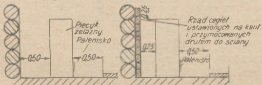
Rys. 141. Izolacja przewodów dymnych: a) przewód dymny w pobliżu ścian drewnianych bez izolacji; b) przewód dymny w pobliżu ścian drewnianych z zastosowaniem izolacji; c) przepuszczenie przewodu dymnego przez ścianę drewnianą z izolacją ziemną; d) to samo z izolacją z piaskownicy
