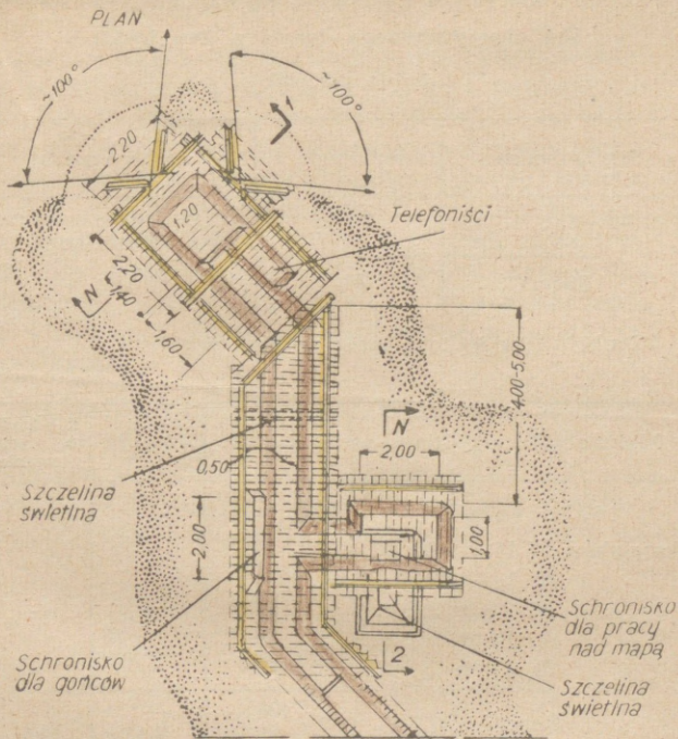
PRZEKRÓJ N-1
