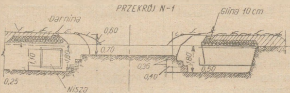
Rys. 39. Stanowisko dla 76 mm dział artylerii dywizyjnej z wycinkiem ostrzału ograniczonym (do 100^{\circ} )
