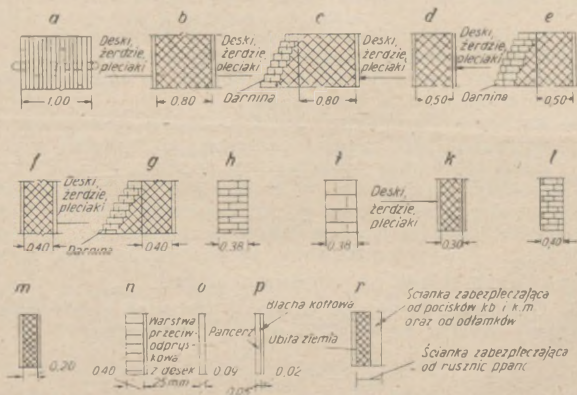
Rys. 1-b. Warstwy ochronne dla ścian typu lekkiego (od pocisków rusznic ppanc i serii ckm): a) okrągłaki sosnowe na poprzek; b) i c) ubity torf; d) i e) ubita ziemia, glina, ziemia gliniasto piaszczysta; f) i g) ubita ziemia; h) cegła na zaprawie cementowej; i) kamienie żużlowe na zaprawie cementowej; k) ubity piasek; l) kamienie łamane na zaprawie cementowej; m) ubity żwir z piaskiem; n) elementy żelazobetonowe na zaprawie cementowej; o) blacha kotłowa nr 30; p) blacha pancerna i kotłowa; r) wzmocnienie 16 mm ściany kopuły żelazobetonowej warstwą ziemi o grub. 20 cm
