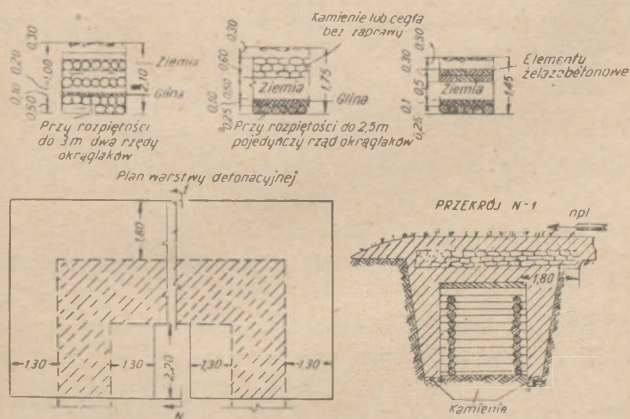
Rys. 5. Warstwy ochronne w budowlach typu wzmocnionego
