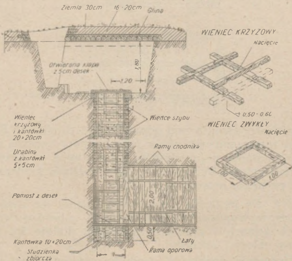
Rys. 180. Zapuszczanie szybu w gruntach sypkich (typ I)
