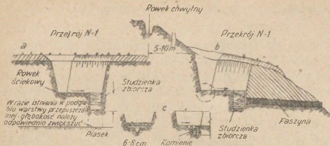
Rys. 65. Odprowadzenie wody z rowów strzeleckich i łączących: a) budowa studzienki zbiorczej w terenie równinnym, b) budowa rowków chwytlnych, studzienki zbiorczej oraz drenowanie na stoku; c) szczegóły budowy rowków.
