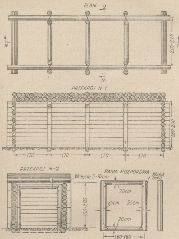
Rys. 151. Rama rozporowa i wzmocnienie szkieletu wieńcówki za pomocą ściągów
