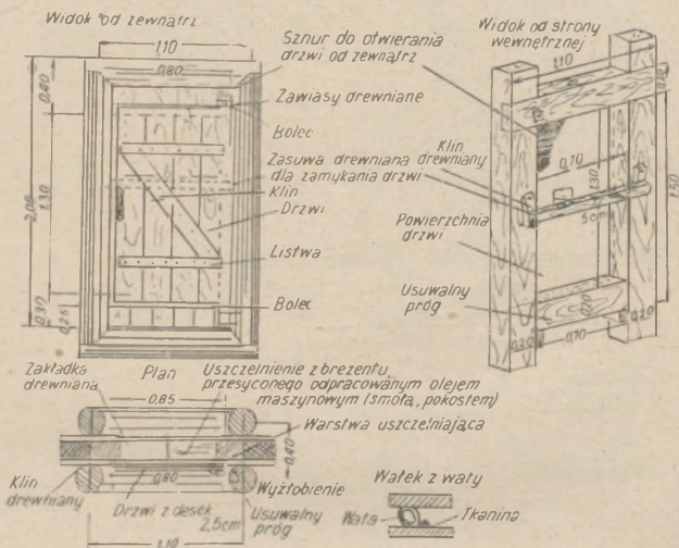
Rys. 132. Drzwi gazoszczelne
