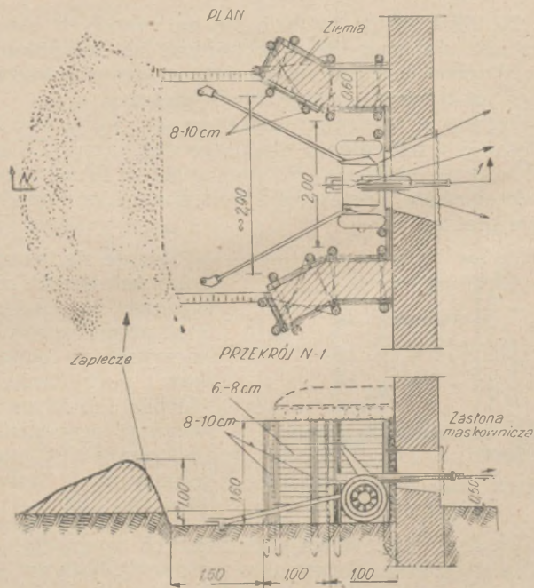
Rys. 83. Wykorzystanie muru dla urządzenia stanowiska działa 45 mm
