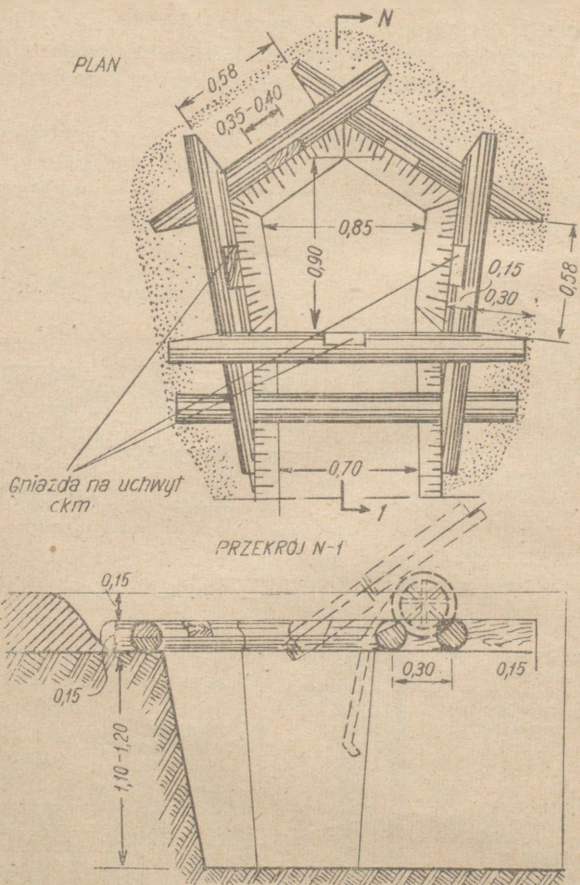
Rys. 32. Stanowisko plot dla ckm, na podstawie Sokołowa, umieszczonego na drewnianym ramie
