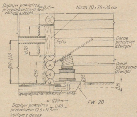
Rys. 133. Instalacja filtro-wentylacyjna typu M-20 w schronie
