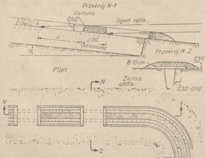
Rys. 60. Poprzecznicę wiszące w rowie łączącym
