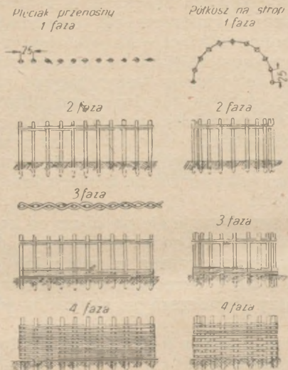
Rys. 147. Wyrób pleciaków
