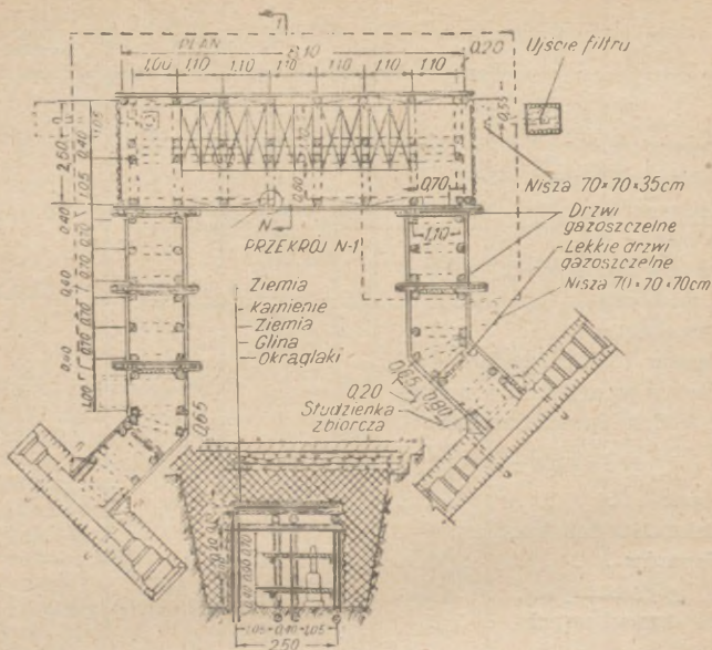
Rys. 77. Schron wykopowy, konstrukcji jarzmowej typu wzmocnionego (lub ciężkiego) na 20 ludzi
