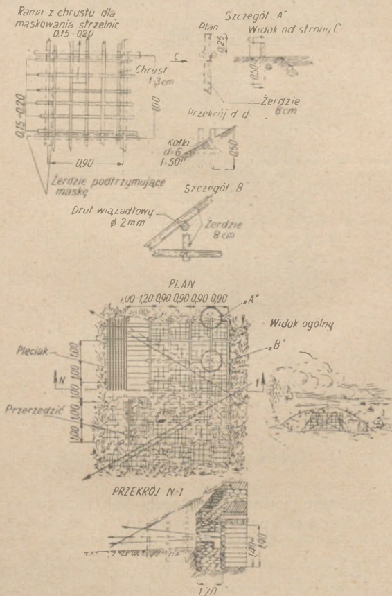
Rys. 122. Maskowanie strzelnicy tarczą nieruchomą
