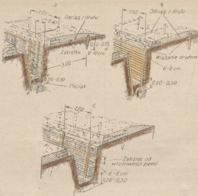
Rys. 63. Odziewanie ścian rowów strzeleckich lub łączących: a) odziewanie pleciakami; b) odziewanie żerdziami całkowite; c) odziewanie żerdziami częściowe
