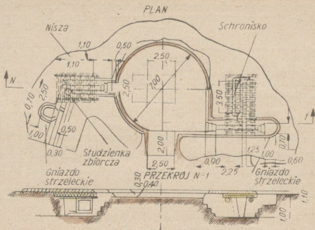
Rys. 38. Stanowisko dla 76 mm działa art. dywizyjnej (stanowisko dla ostrzału wkoło)
