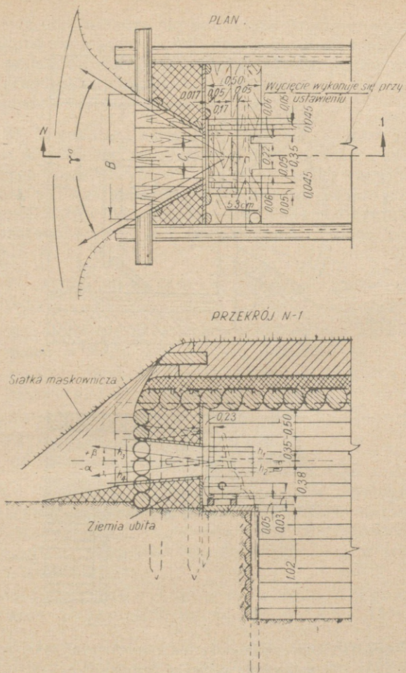
Rys. 116. Umocowanie ckm na nieruchomym stole, z opuszczeniem uchwyty
