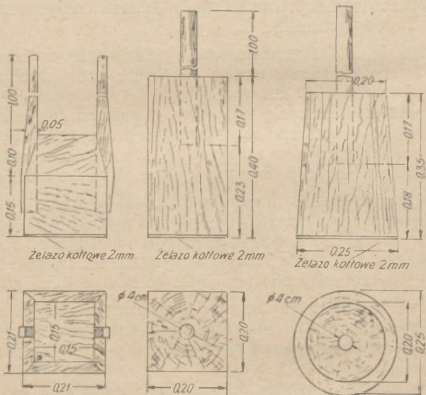
Rys. 145. Typy ubijaków
