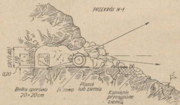
Rys. 107. Przystosowanie pieczary na stanowisko ogniowe dla dział 76 i 45 mm (wymiarzy w nawiasach podane dla dział 45 mm)
