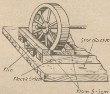
Rys. 117. Szczegół umocowania kółka ckm do stołu
