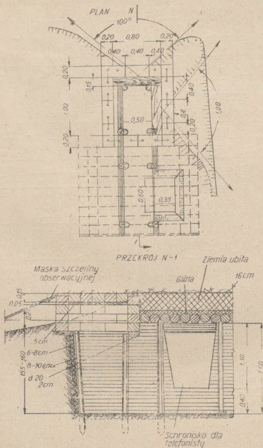
Fys. 43. Żelazobetonowy punkt obserwacyjny, składany, typu przeciw odłamkom (druga szczelina obserwacyjna jest zaznaczona linią wykropkowaną)
