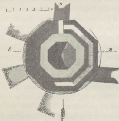
Przekrój poziomy baszty zamkowej w Rawie.
