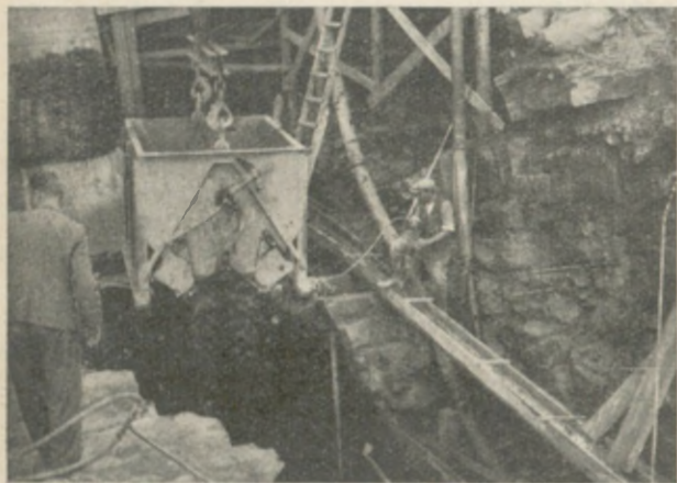
Budowa zapory zbiornika retencyjnego w Porąbce. Wylewanie betonu na budowę fundamentów zapory.
