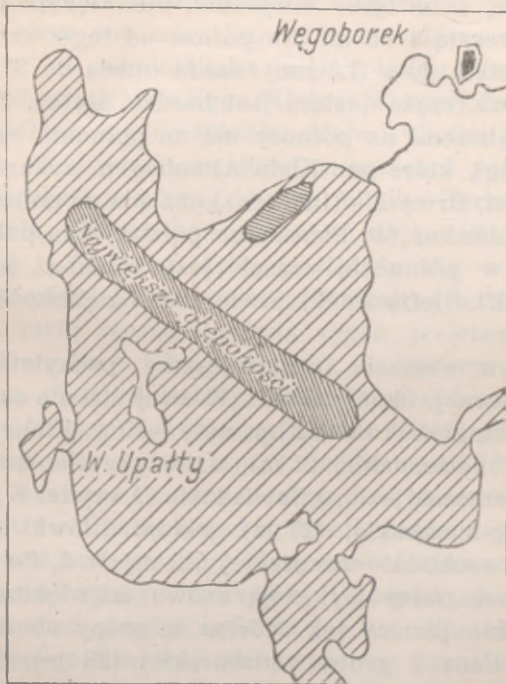
Pas największych głębokości w jez. Mamry.
