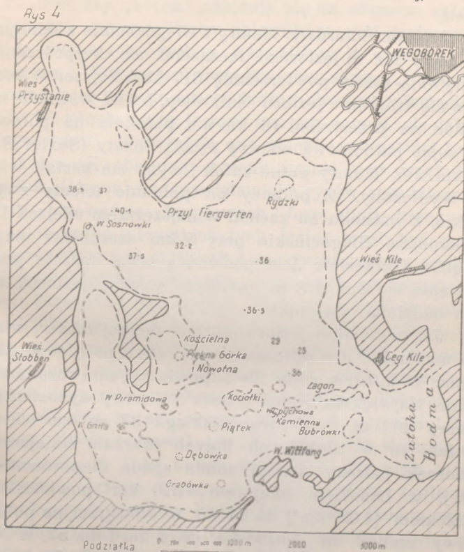
Ukształtowanie dna w jez. Mamry. Linia przerywana oznacza głębokość — 3 m.
