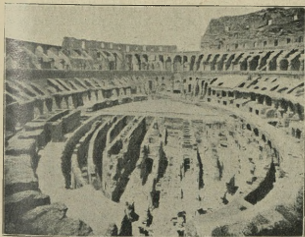
206. Arena w Kolosseum. Podziemia i fundamenty.
