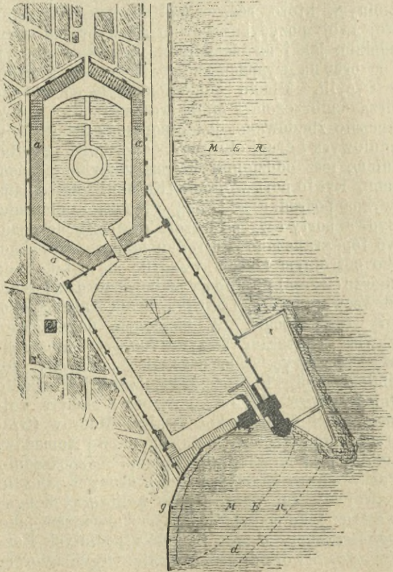
67. Plan portu Kartaginy. Według Daux'a.
