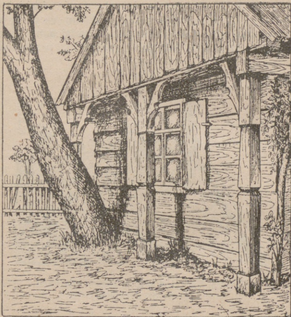
Ryc. 14. Chałupa w Jorkowie (pow. Węgorborski) z podcieniami.
