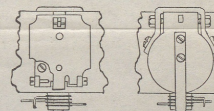
Rys. 5. Mechanizm klapy widziany z boku, z przodu i z tyłu.
