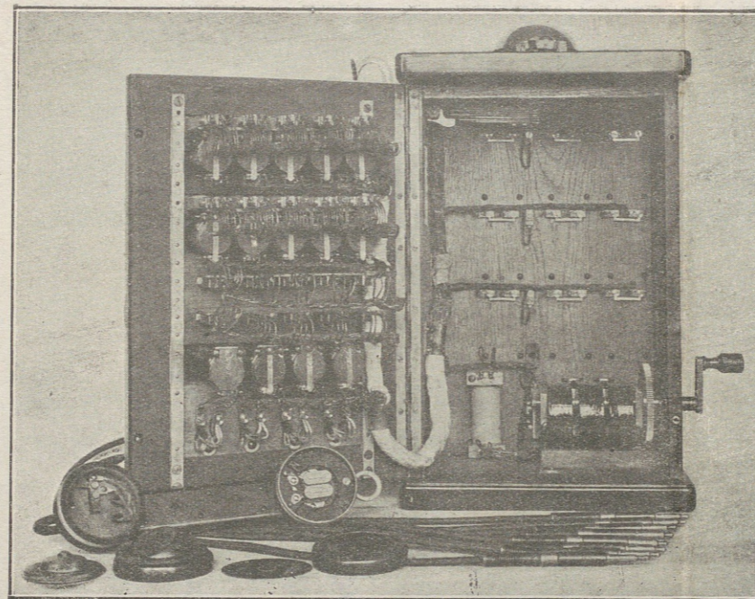
Rys. 3. Wnętrze urządzenia łącznicy MB-05 na 10 połączeń.
