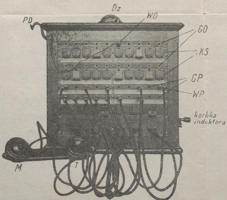
Rys. 2. Łącznica BM-05 na 20 połączeń.
