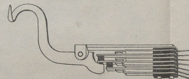
Rys. 6. Przełącznik dźwigniowy.
