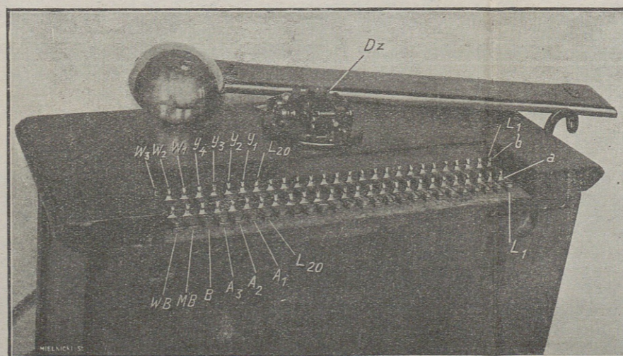
Rys. 7. Zamki zewnętrzne łącznicy BM-05 i dzwonek.
