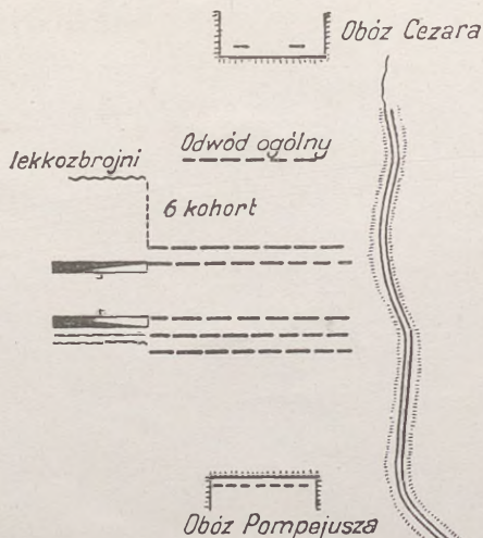
SCHEMAT SZYKÓW BOJOWYCH W BITWIE POD PHARSALUS W R. 48 PRZED CHR.
