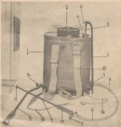
Rys. 3. Rozpylacz „Ama”.
