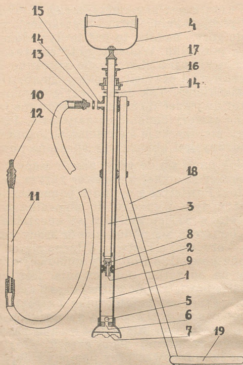
Rys. 5. Hydropult w przekroju schematycznym.
