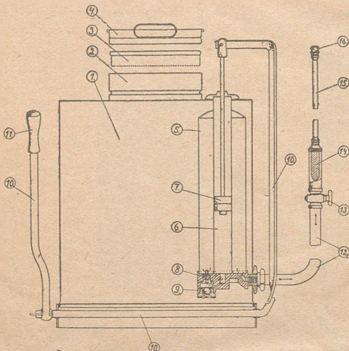
Rys. 4. Rozpylacz „Ama” w przekroju schematycznym.
